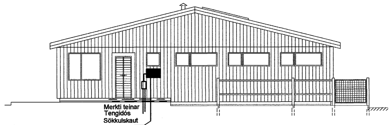
Útlit Norður mkv. 1:100
