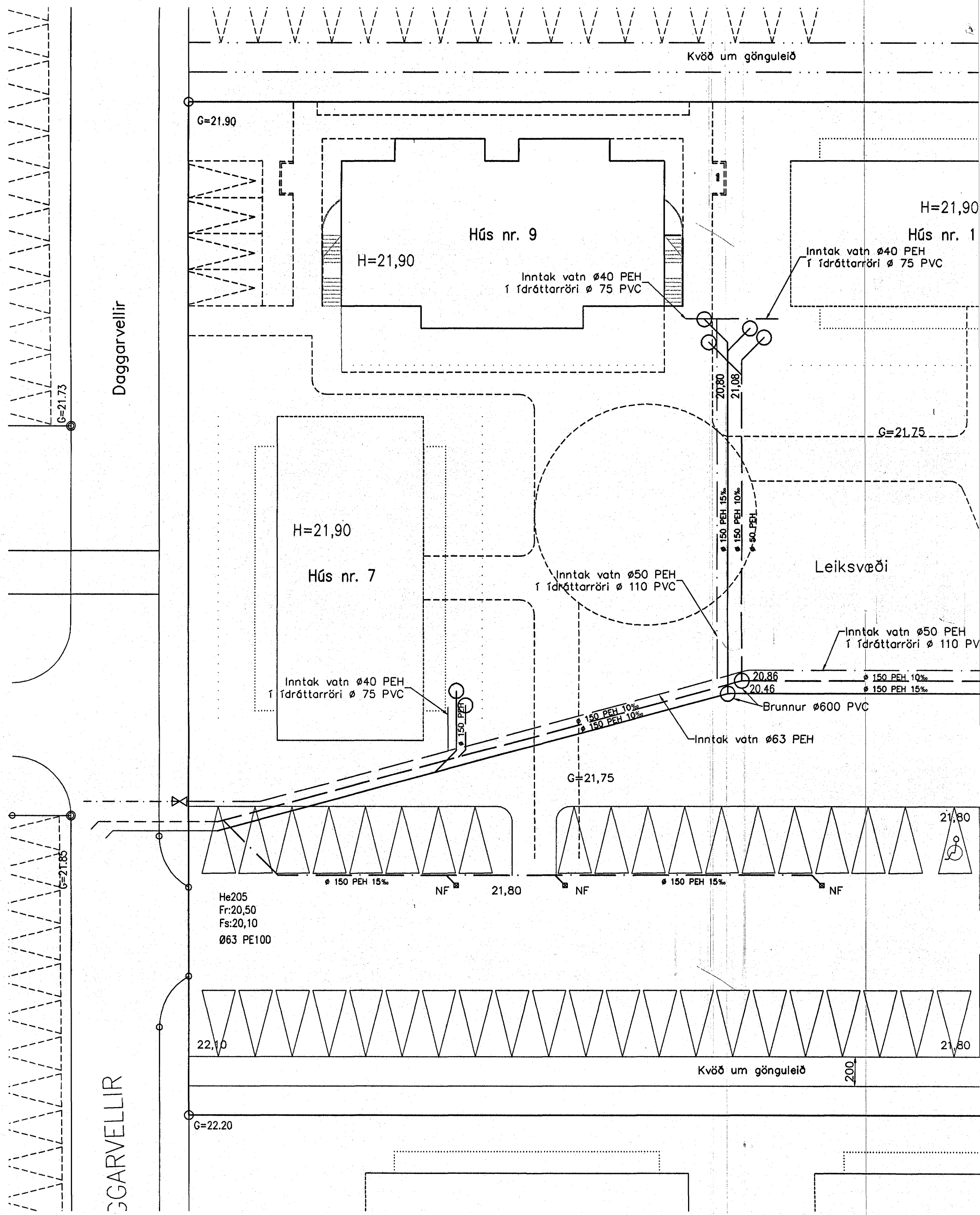
Afstöðumynd, 1:200
