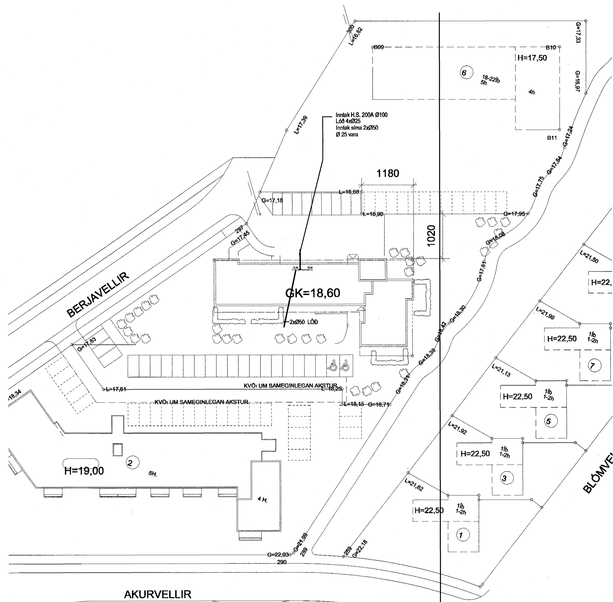
AKURVELLIR AFSTÖÐUMYND, MKV. 1:500
