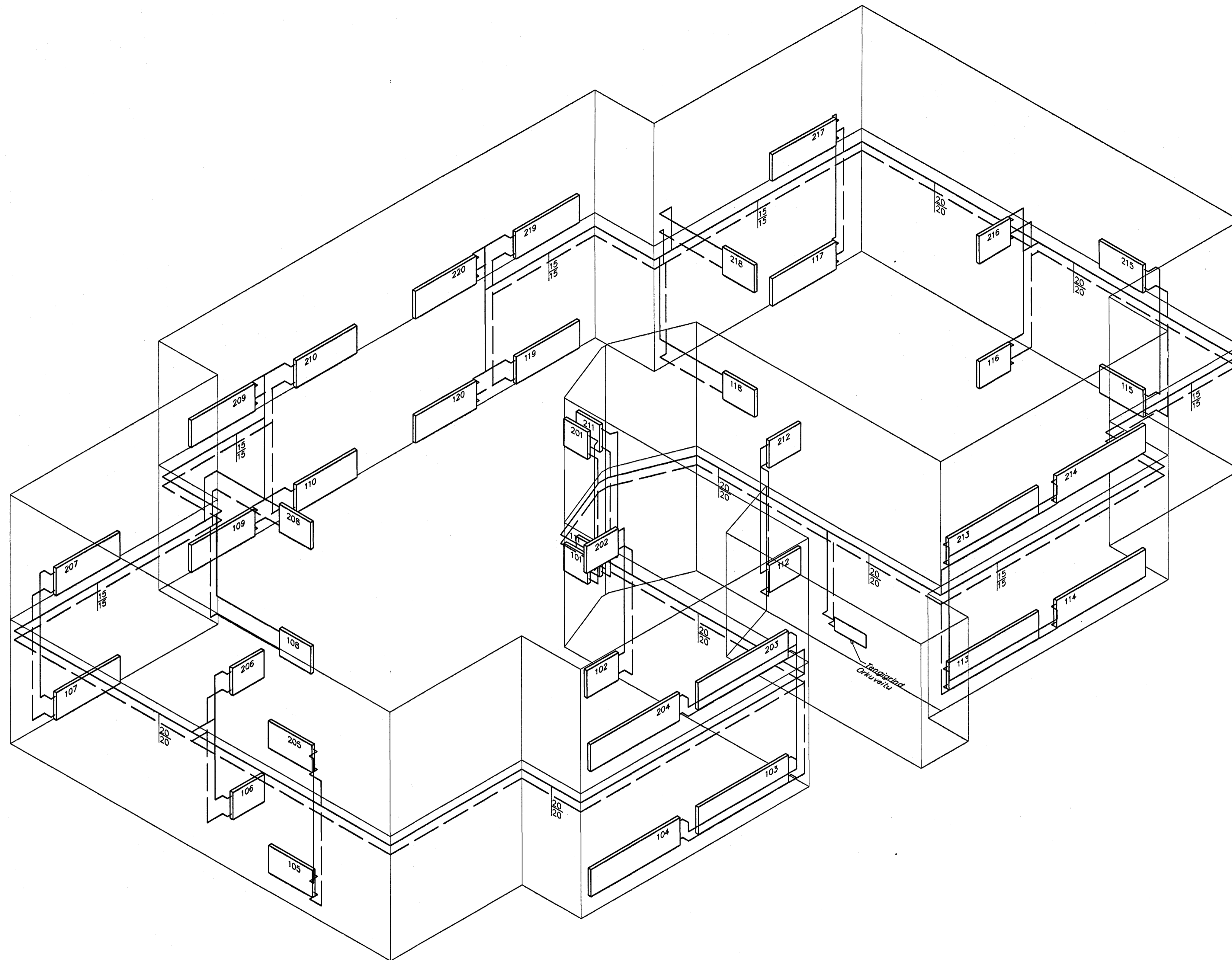
Hitalagnir, Rúmmynd, 1:50
