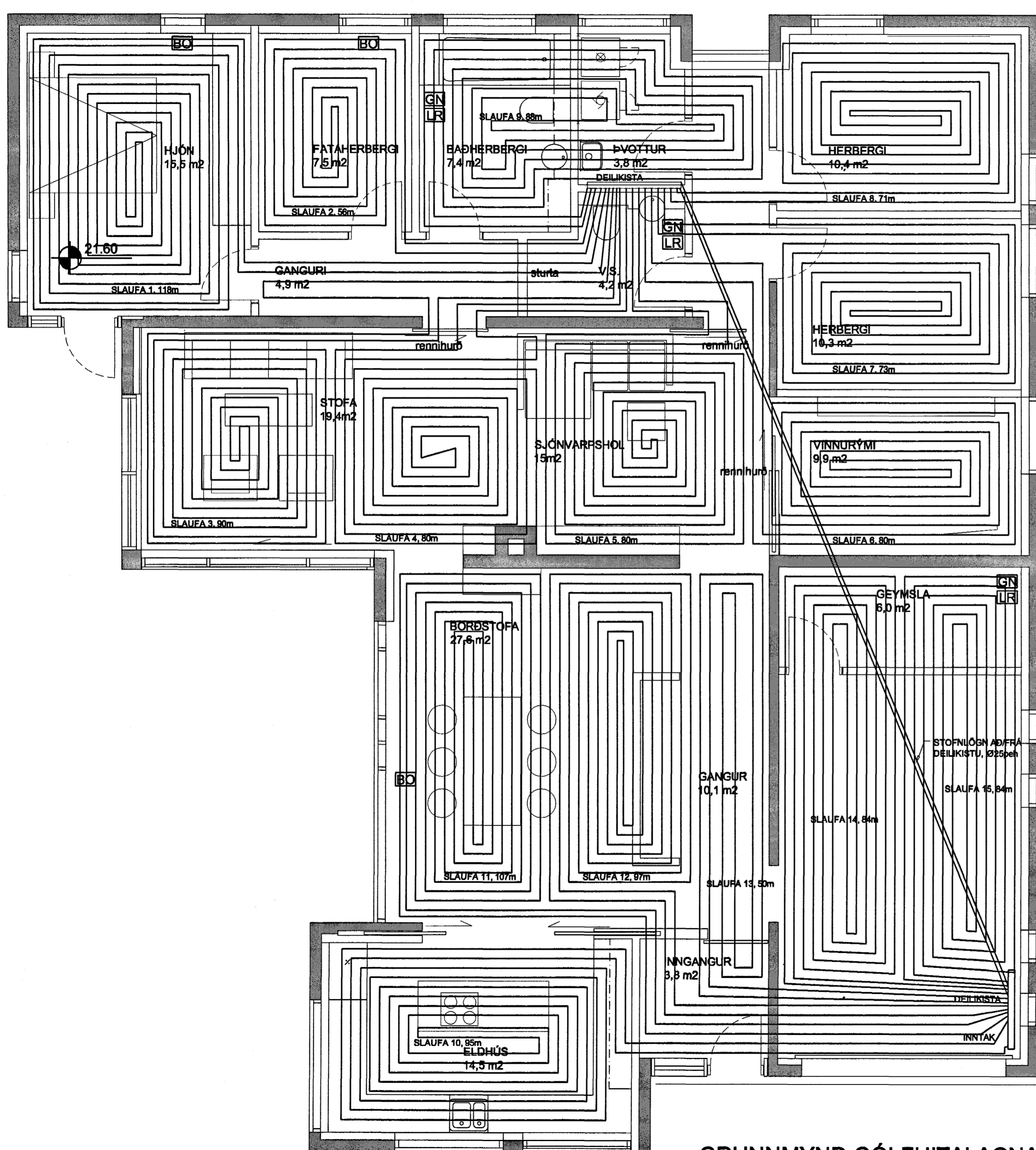
GRUNNMYND GÓLFHITALAGNA, 1:50
