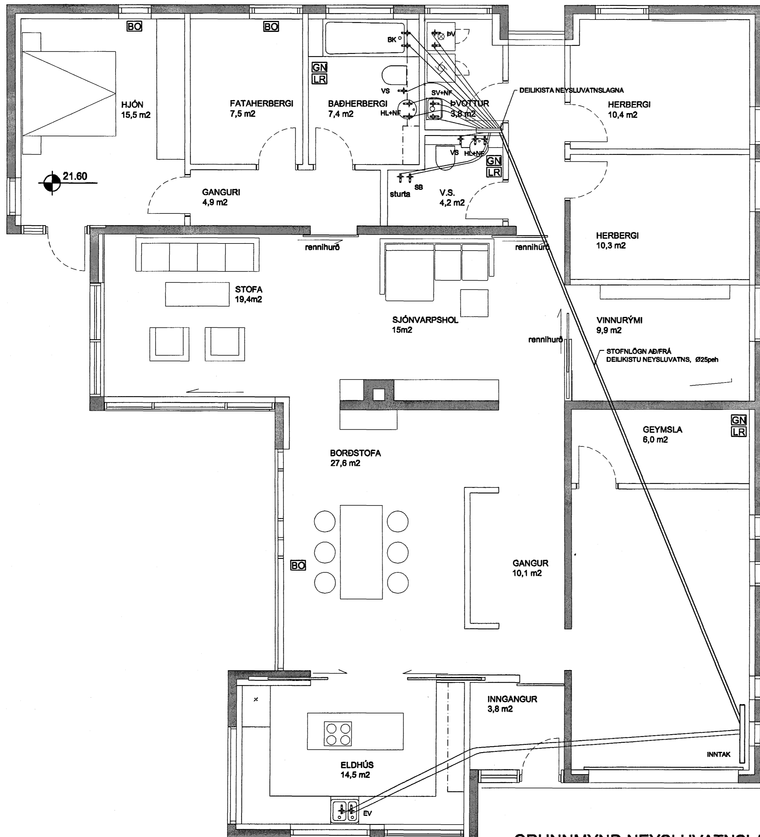
GRUNNMYND NEYSLUVATNSLAGNA, 1:50
