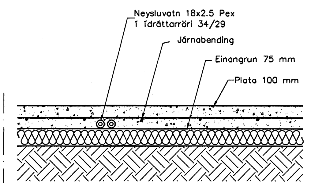
Neysluvatnslagnir, Snið í botnplötu. 1:10
