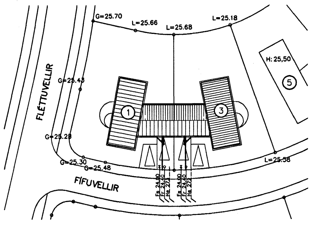
Afstöðumynd, 1:500
