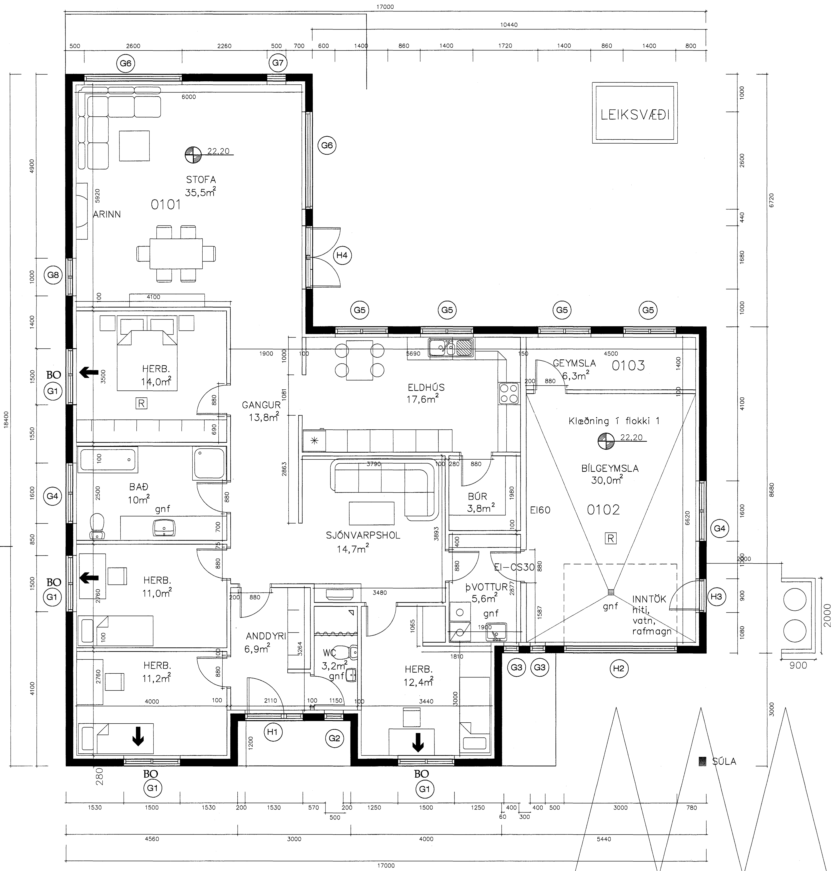
Mkv. 1:50 – GRUNNMYND
