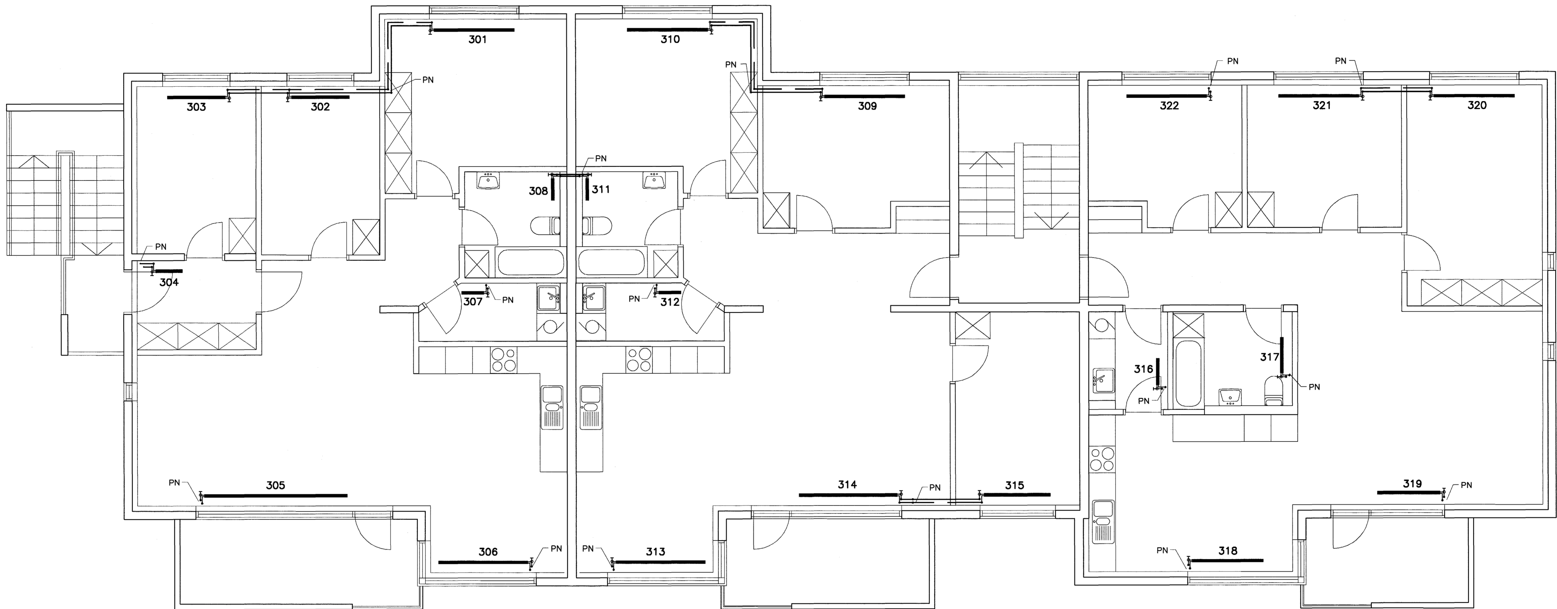
GRUNNMYND 3.HÆÐ. 1:50
