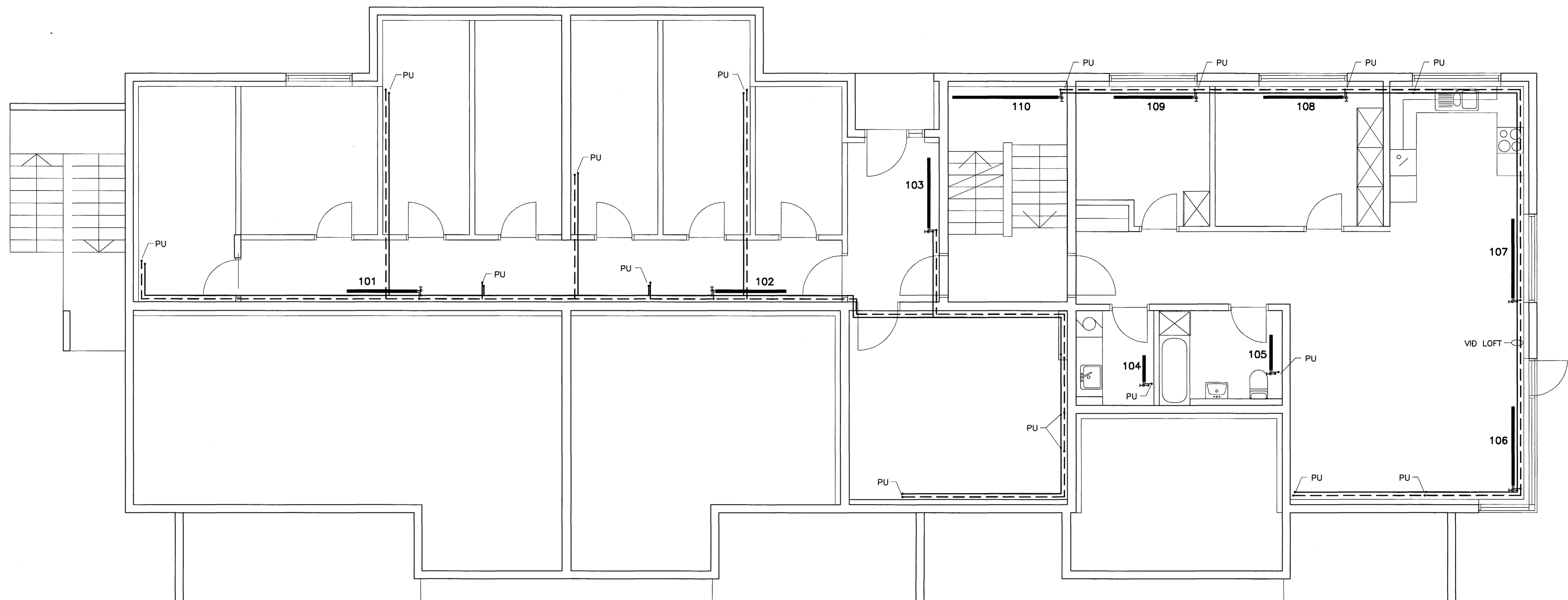
GRUNNMYND 1.HÆÐ. 1:50
