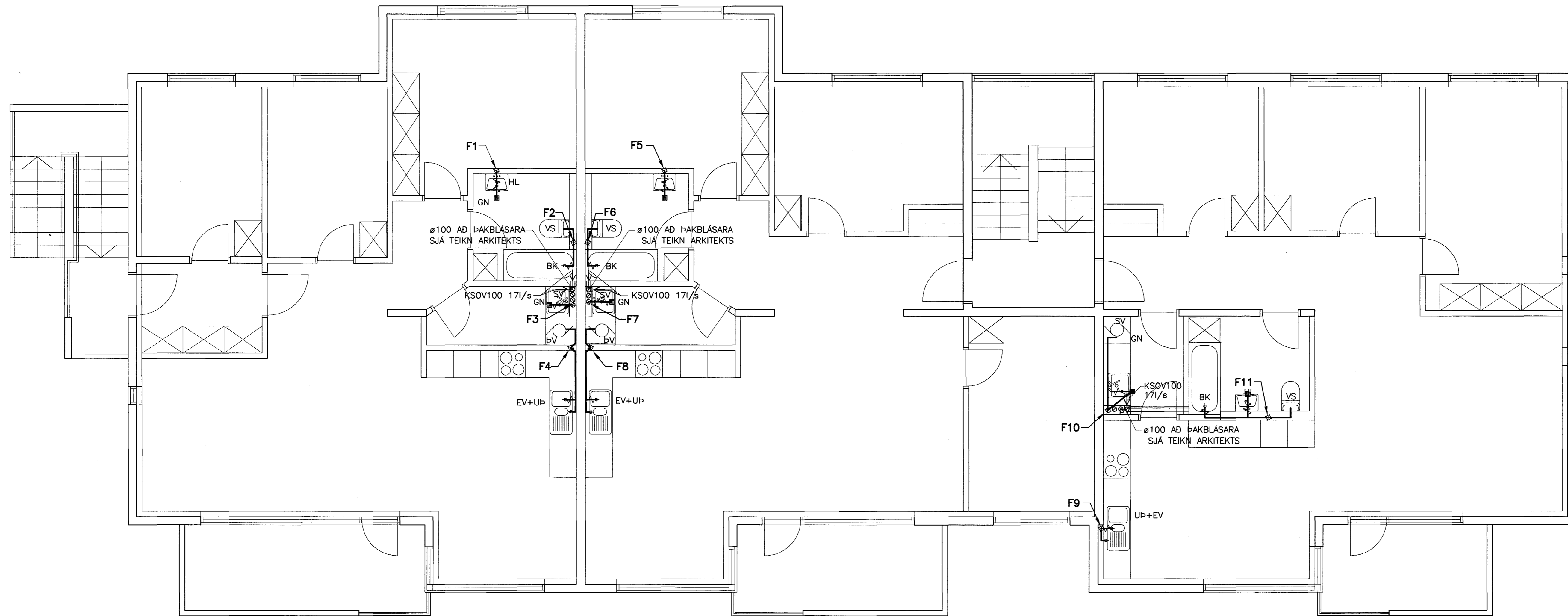
GRUNNMYND 2.HÆÐ. 1:50
