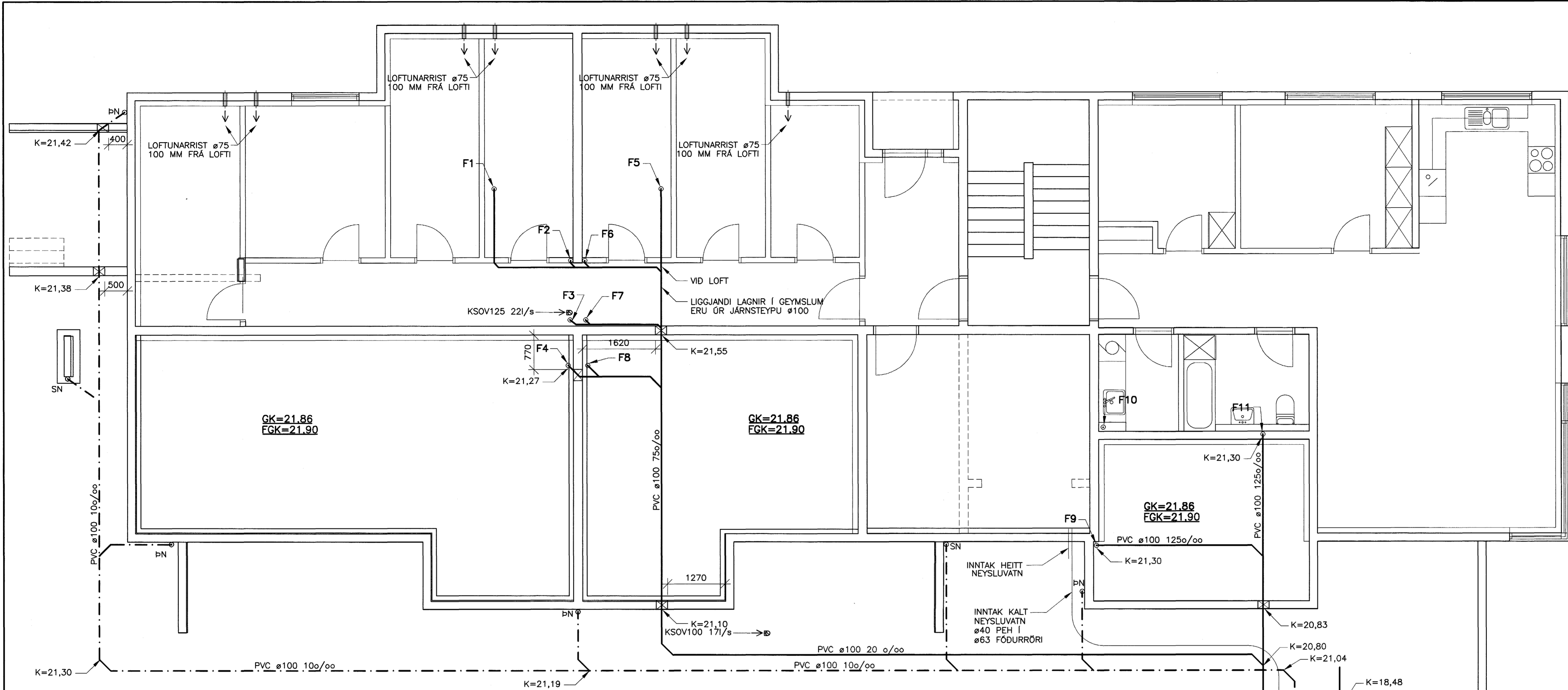
GRUNNLAGNIR GRUNNMYND. 1:50
