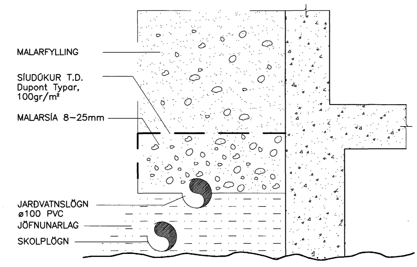
FRÁGANGUR JARDVATNSLAGNA ÚR PVC 1:10
