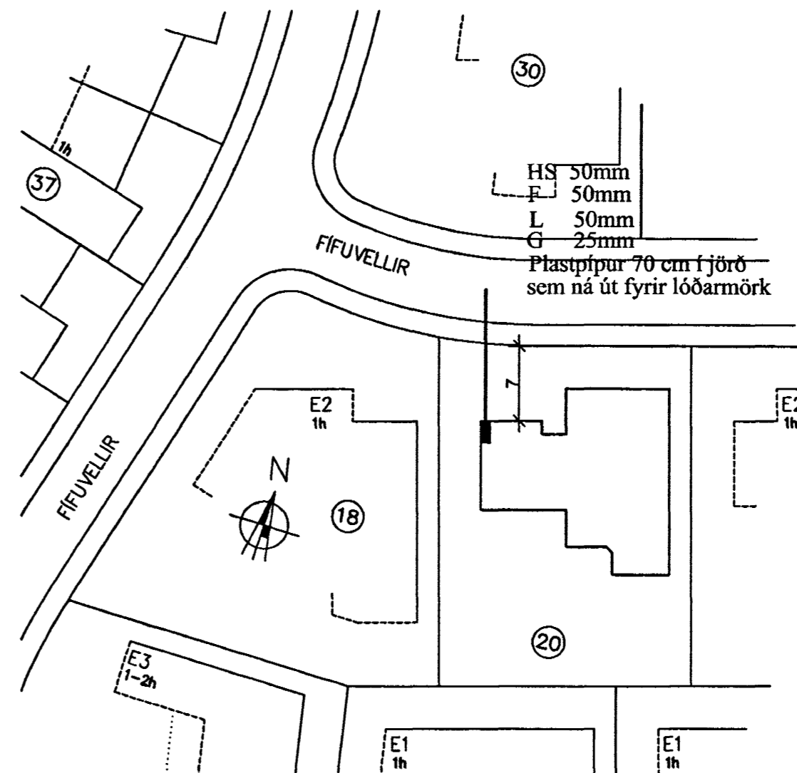
Afstöðumynd mkv. 1/500
