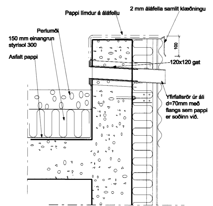
3 DEILI 1:10 Deili í þakbrún með þakyrfirfalli.
