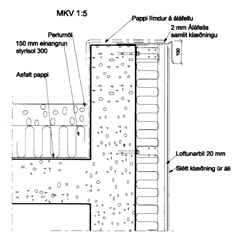
4 DEILI 1:10 36-01 Deili í þakbrún með sléttu áli.
