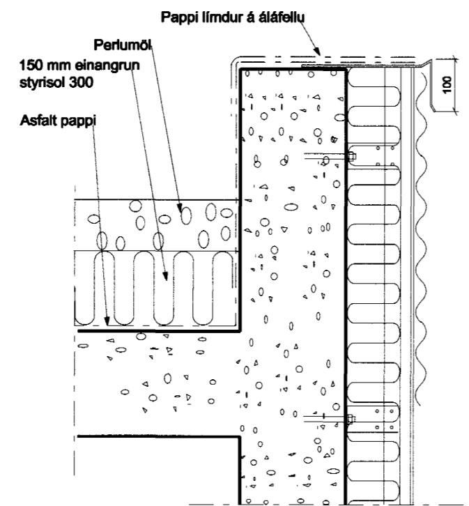
1 DEILI 1:10 20-21 Deili í þakbrún með báruáli
