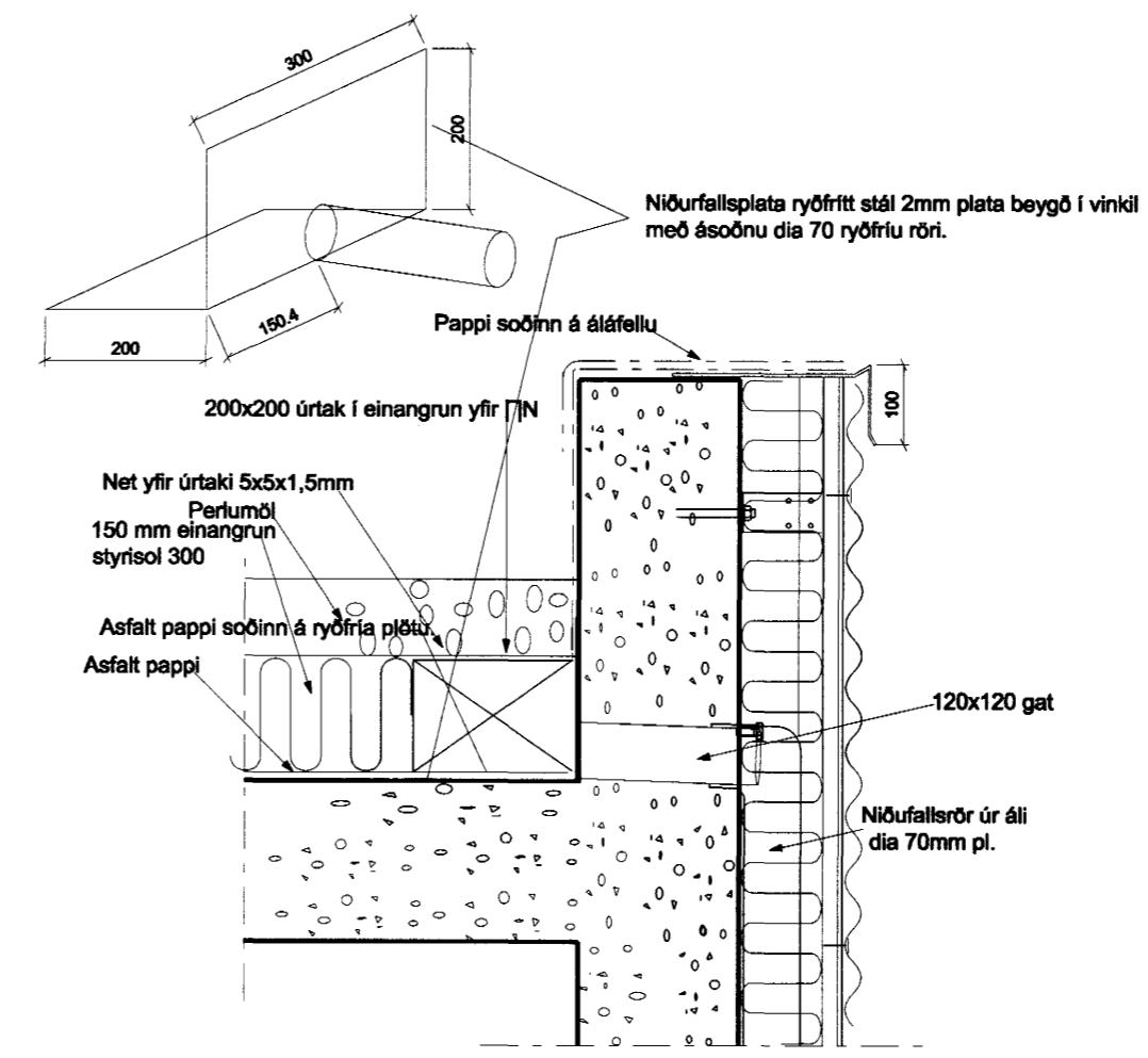
2 DEILI 1:10 Deili í þakbrún með þakniðurfalli.
