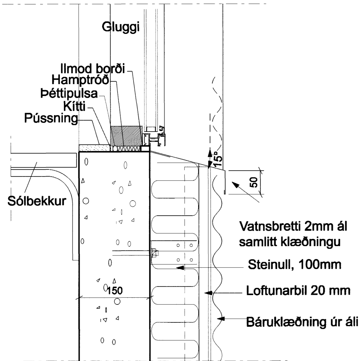
8 DEILI - LÓÐRÉTT 1:5 Deili í glugga í báruáli - undirstykki
