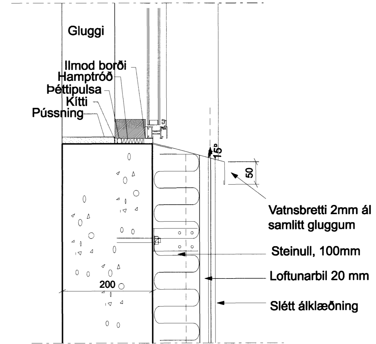
10 DEILI - LÓÐRÉTT 1:5 Gluggi í sléttu áli - undirstykki
