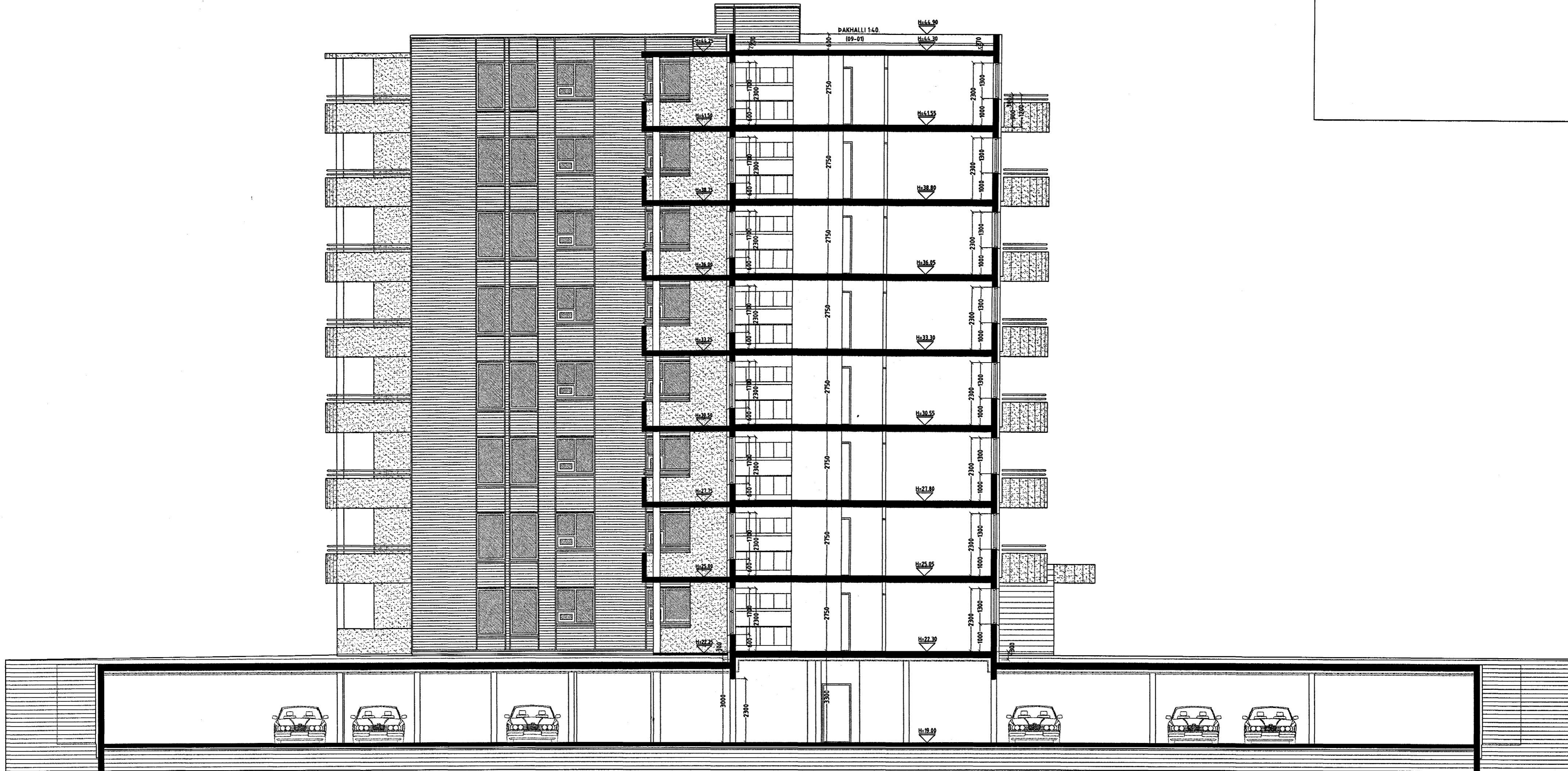
SNID A-A MKV. 1:100.
