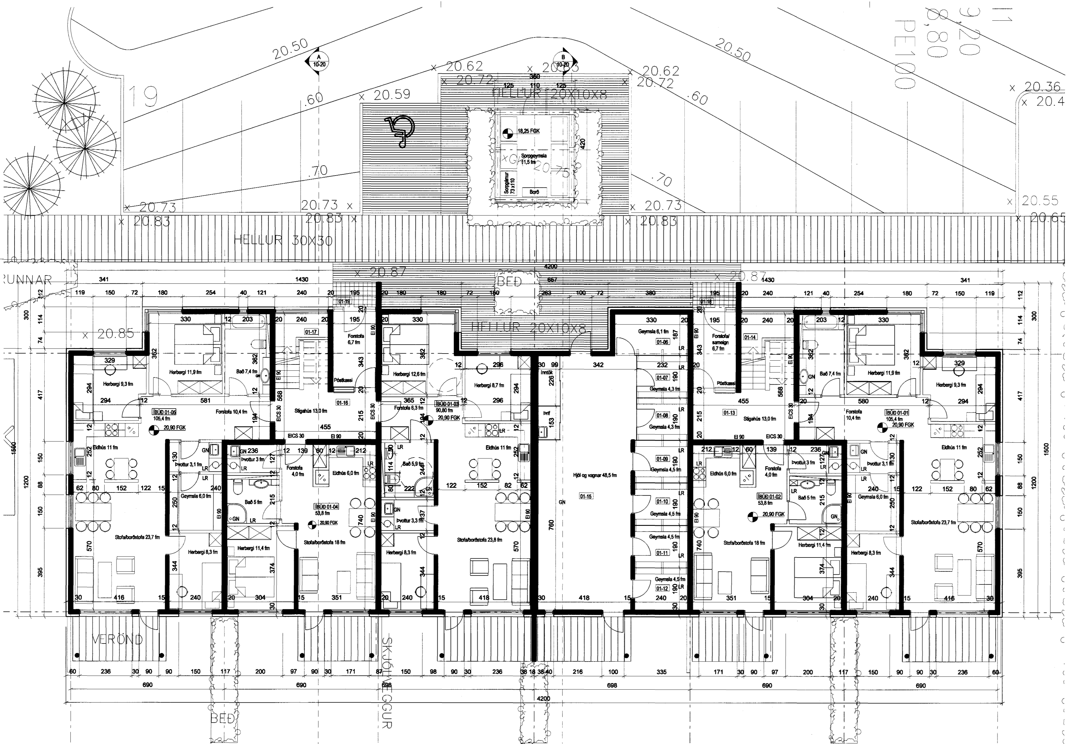
GRUNNMYND 1. HÆÐAR 1:100
