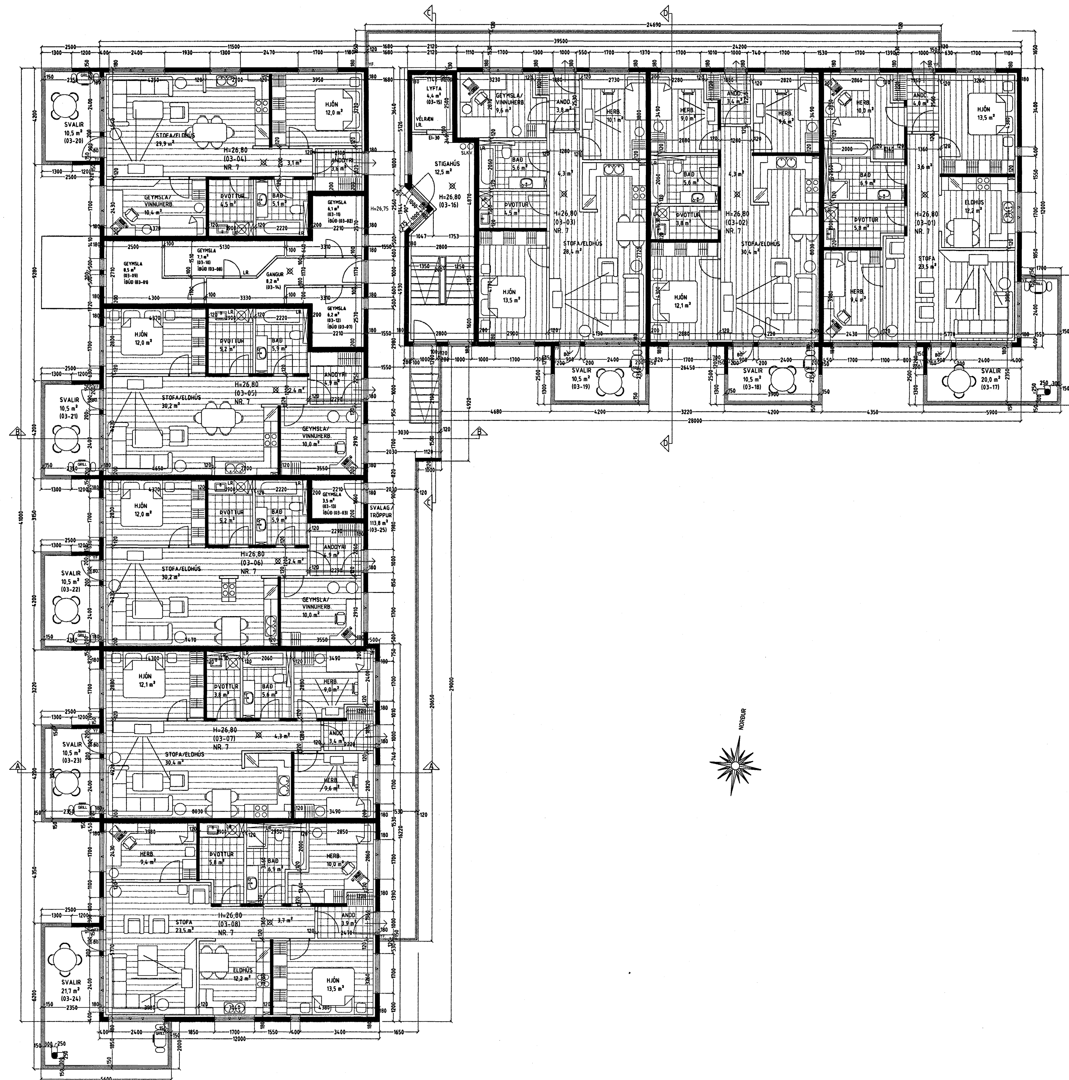
GRUNNMYND 3. HÆÐ MKV. 1:100.
