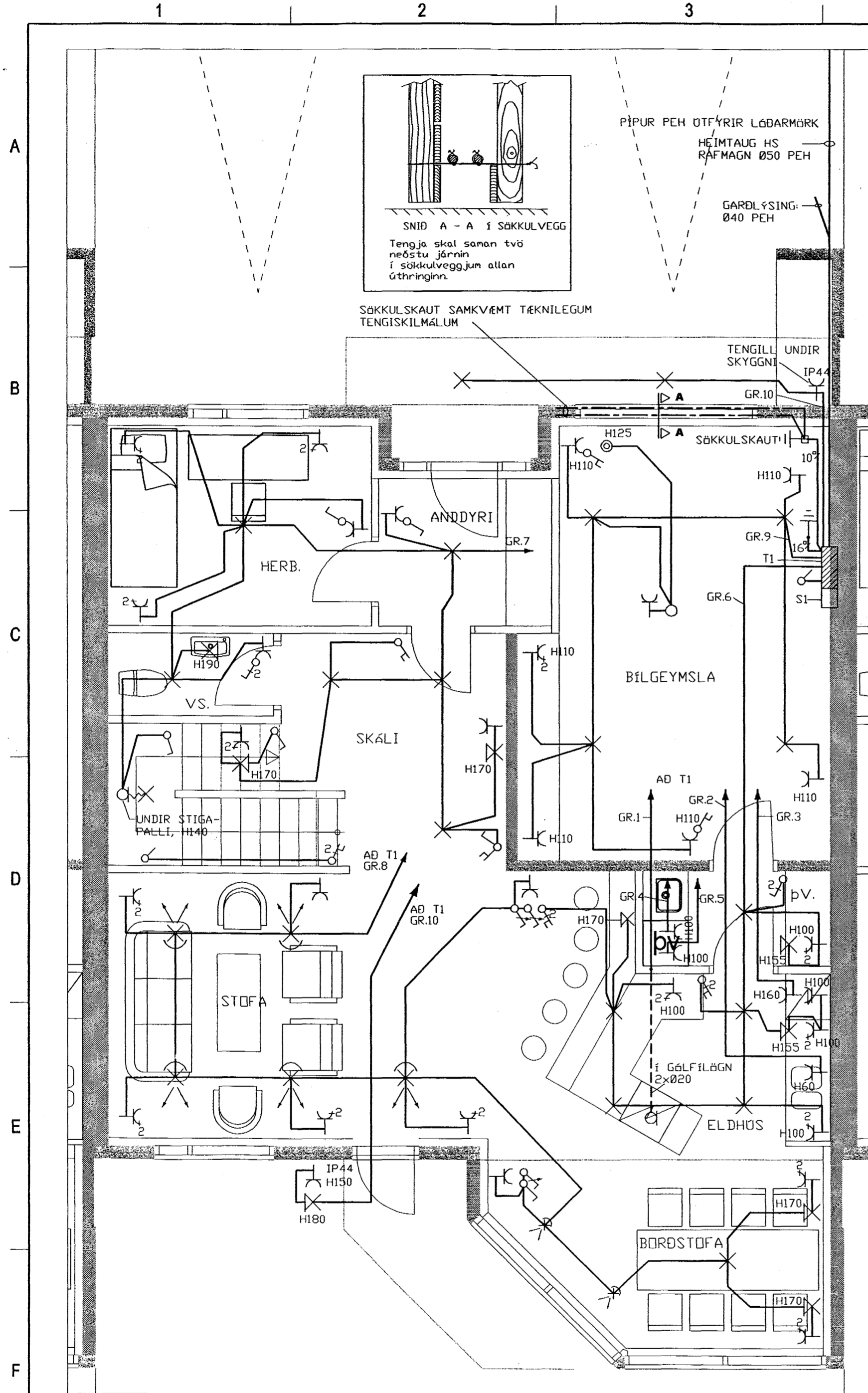
GRUNNMYND 1. HÆÐ
