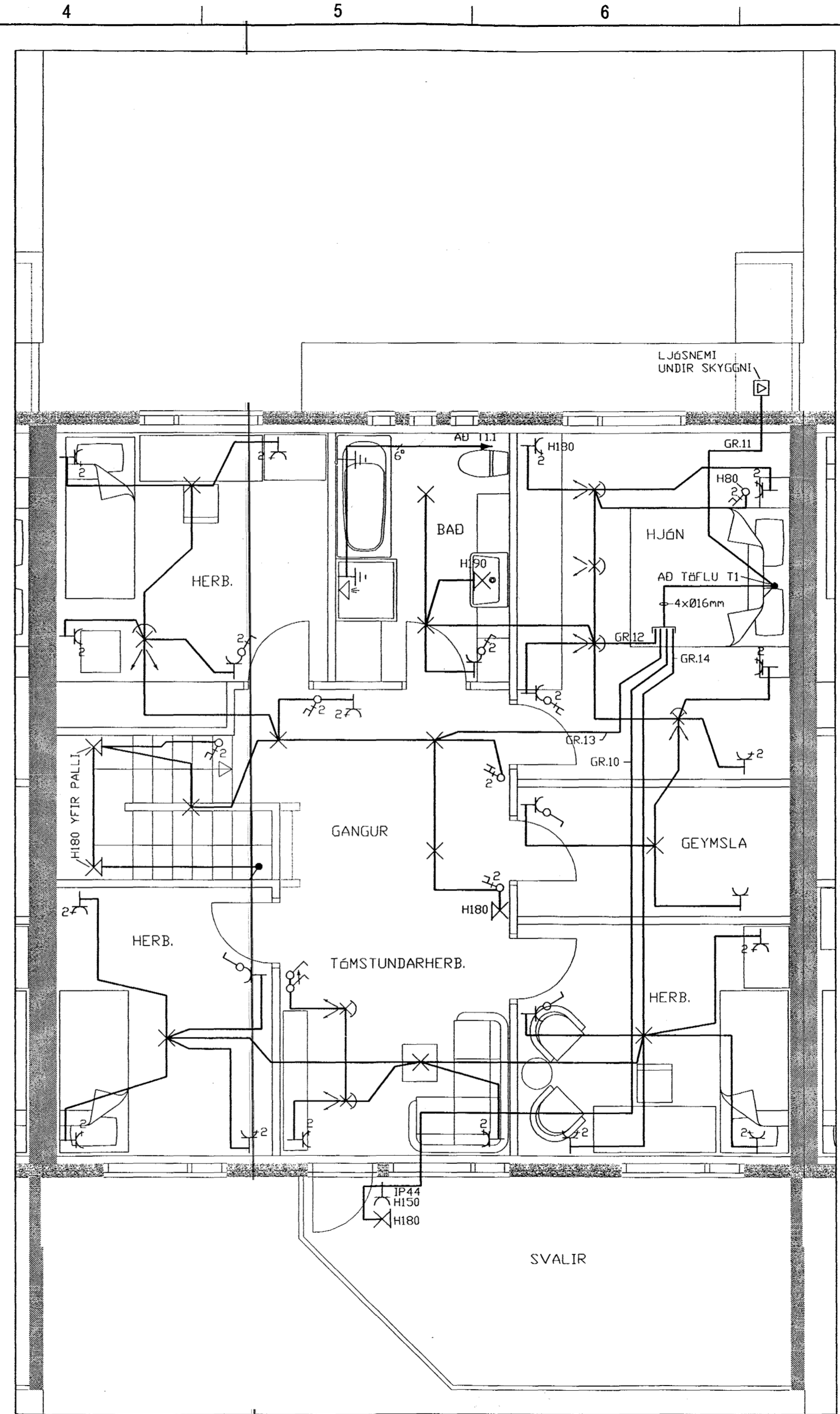
GRUNNMYND 2. HÆÐ
