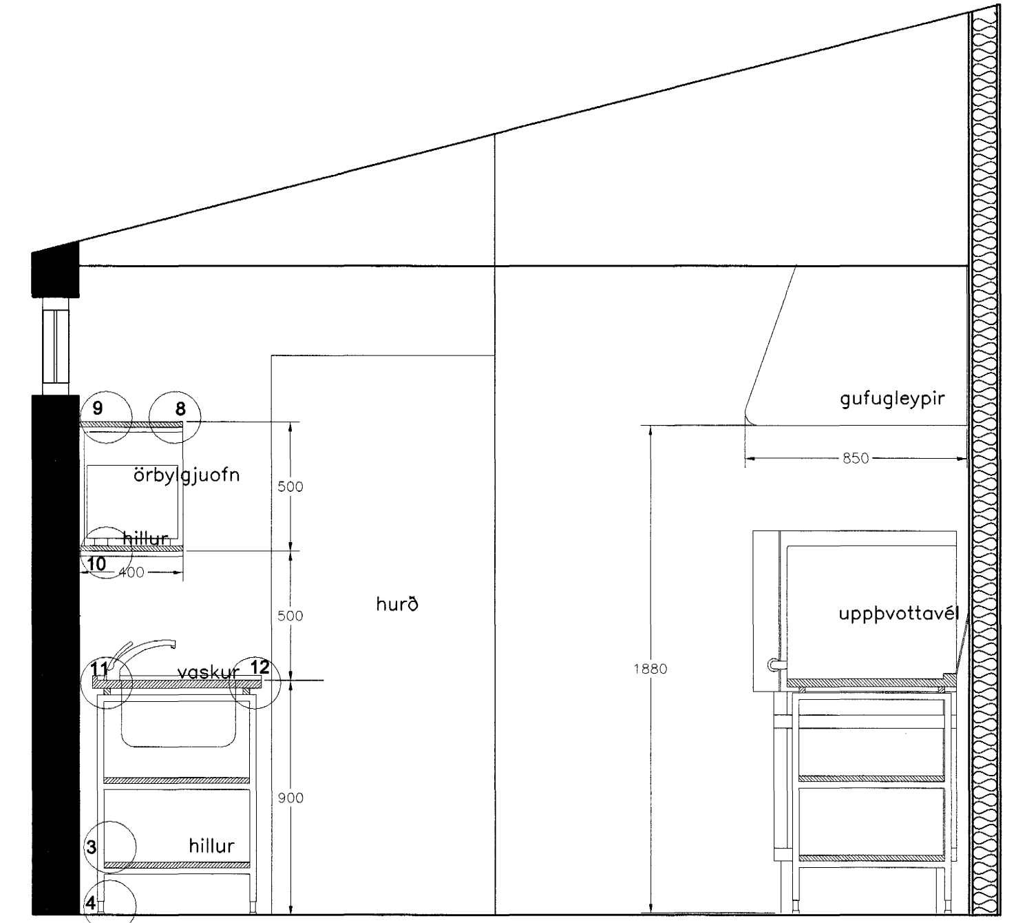
Skurður C - C
