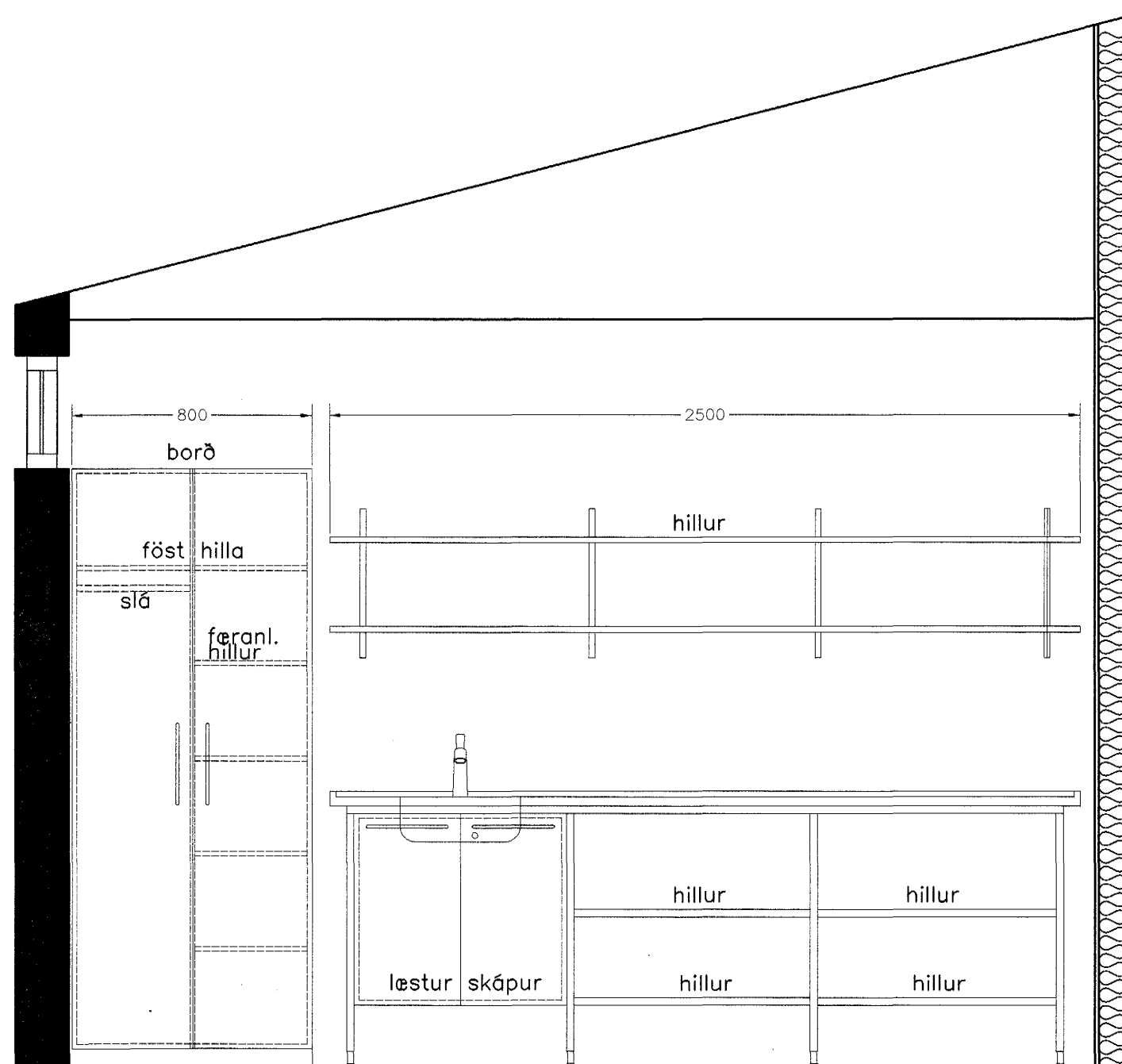
Skurður D - D
