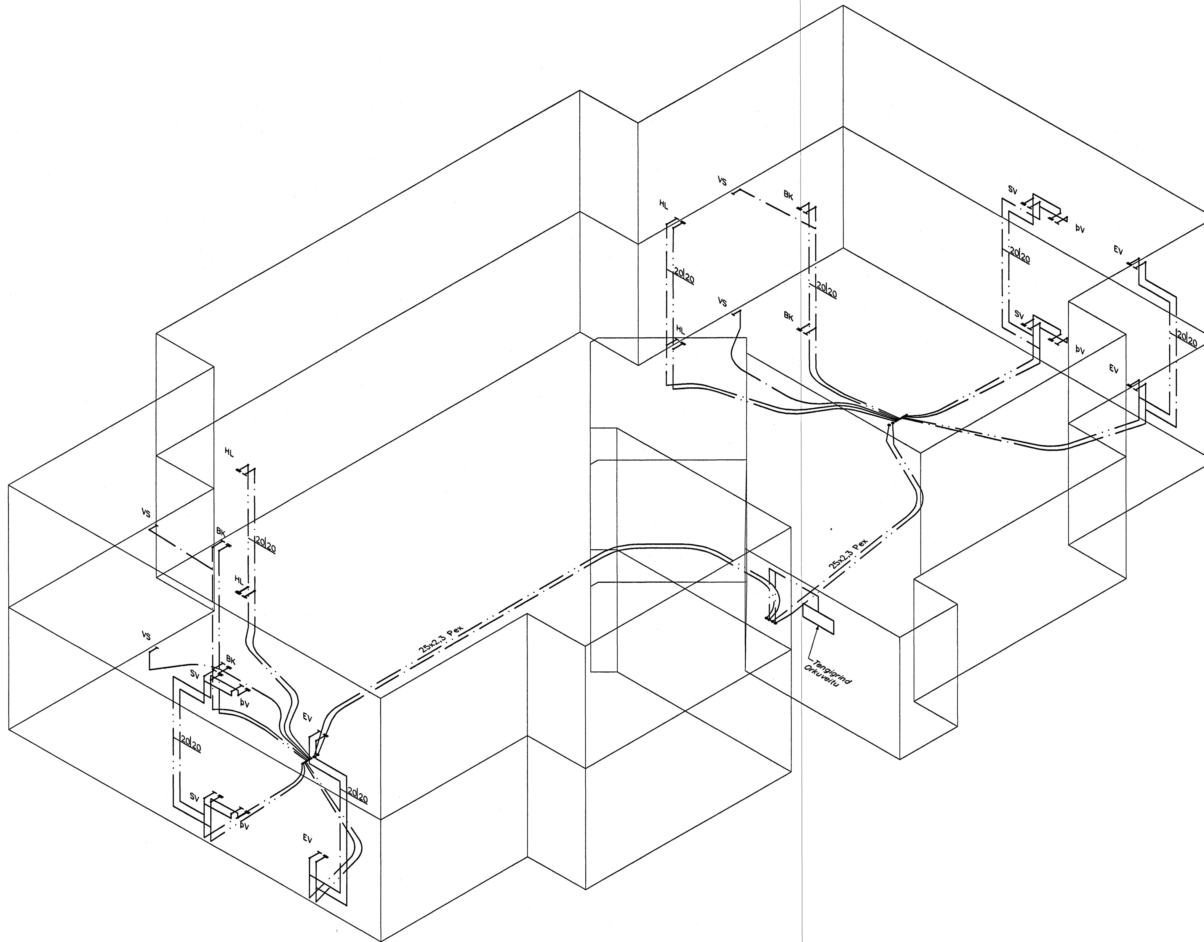
Neysluvatnslagnir, Rúmmynd, 1:50
