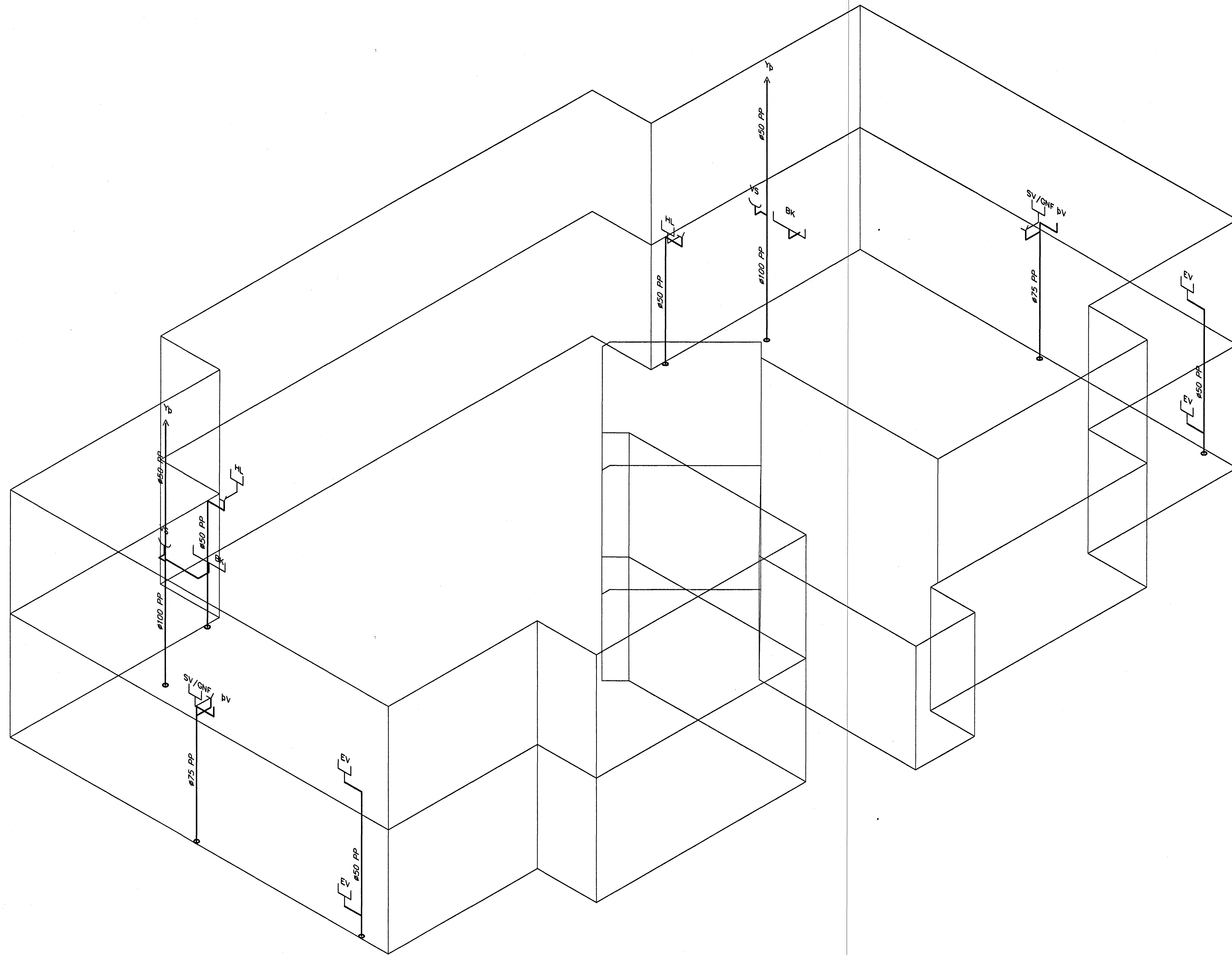
Fráveitulagnir, Rúmmynd, 1:50
