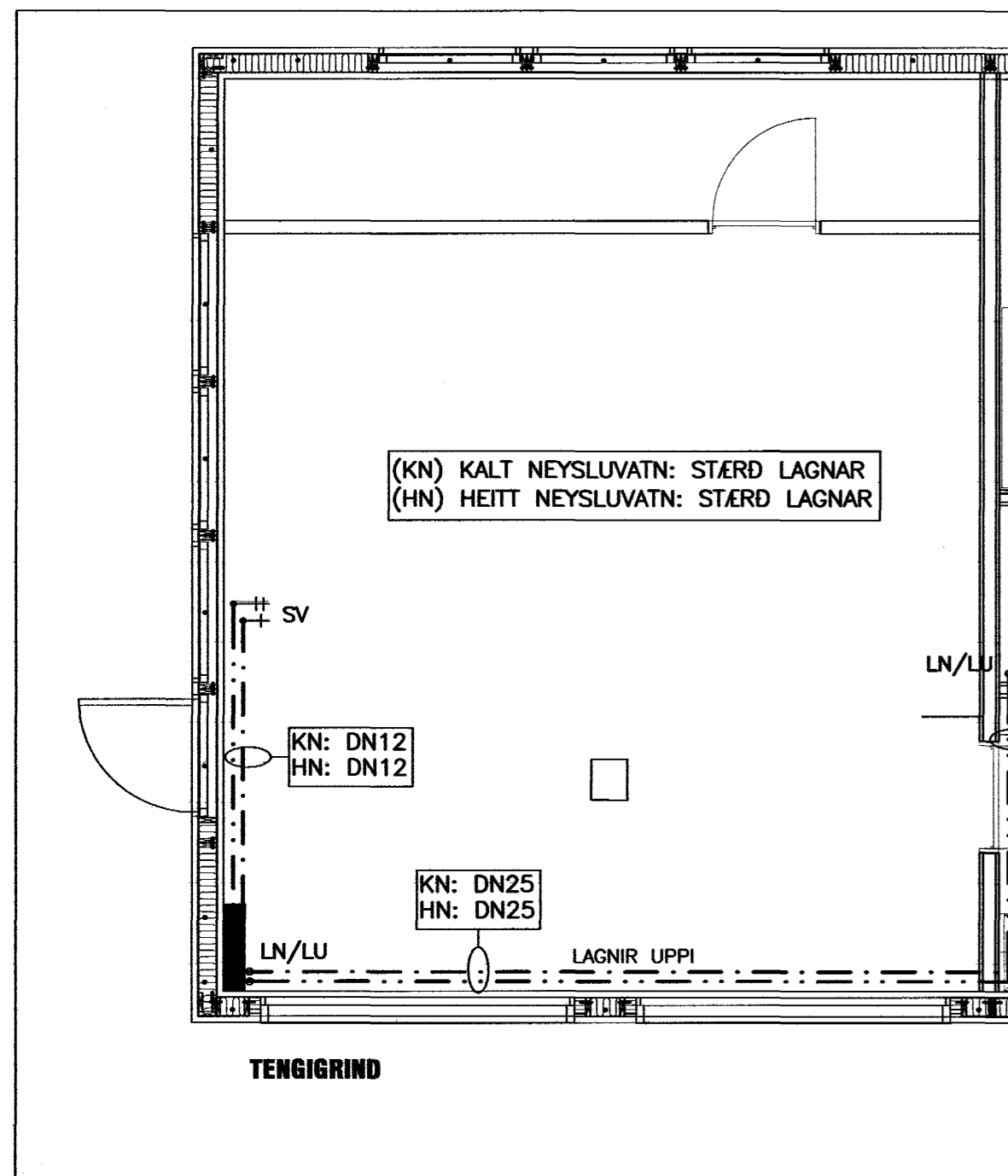
GRUNNMYND HITALAGNA MKV. 1:50
