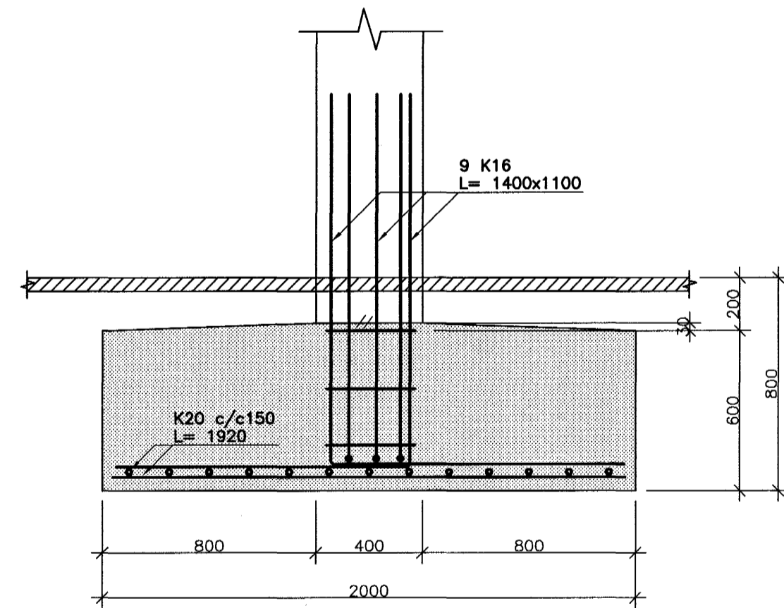
SNID A1 1:20
