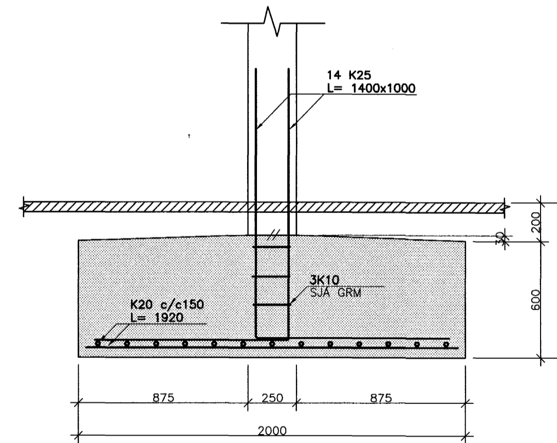
SNID C1 1:20
