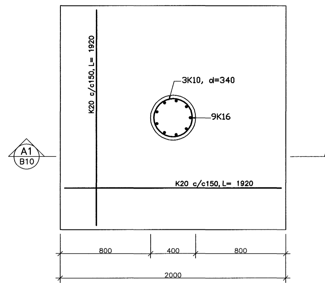
SÓLUFÓTUR A 1:20
