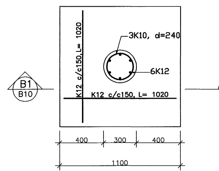
SÓLUFÓTUR B 1:20
