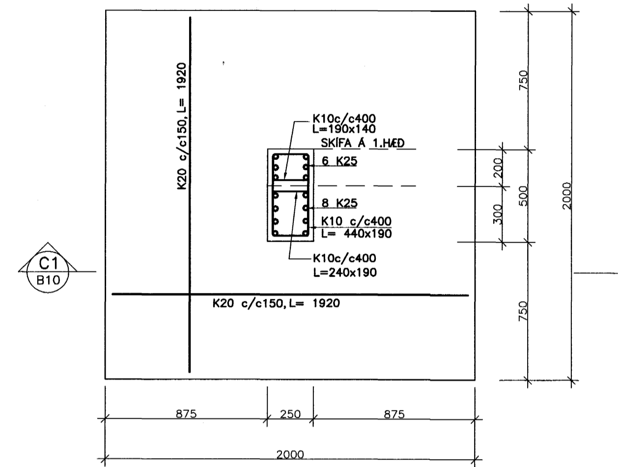
SÓLUFÓTUR C 1:20
