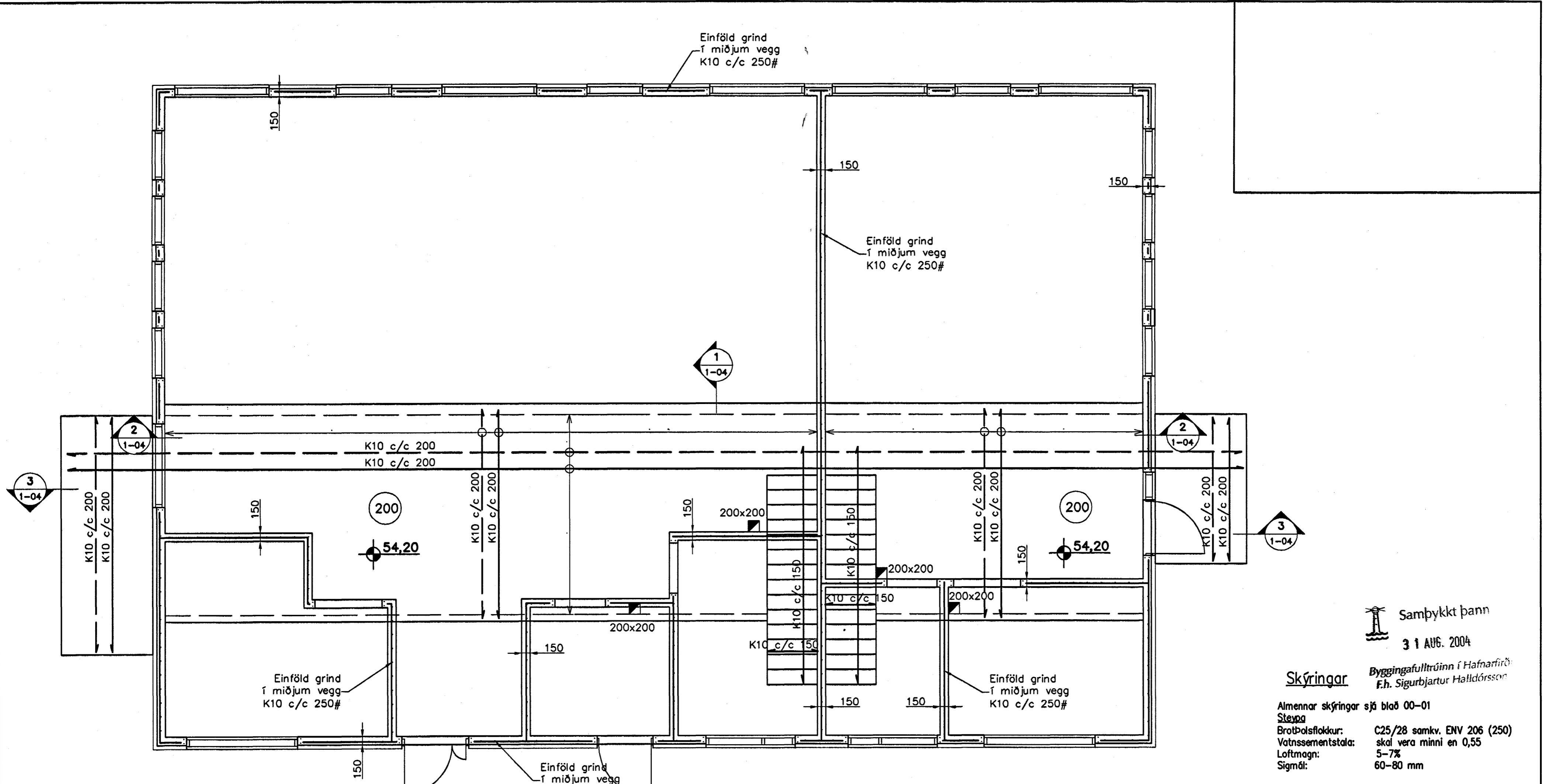
Veggir, Plata, Grunnmynd, 1:50
