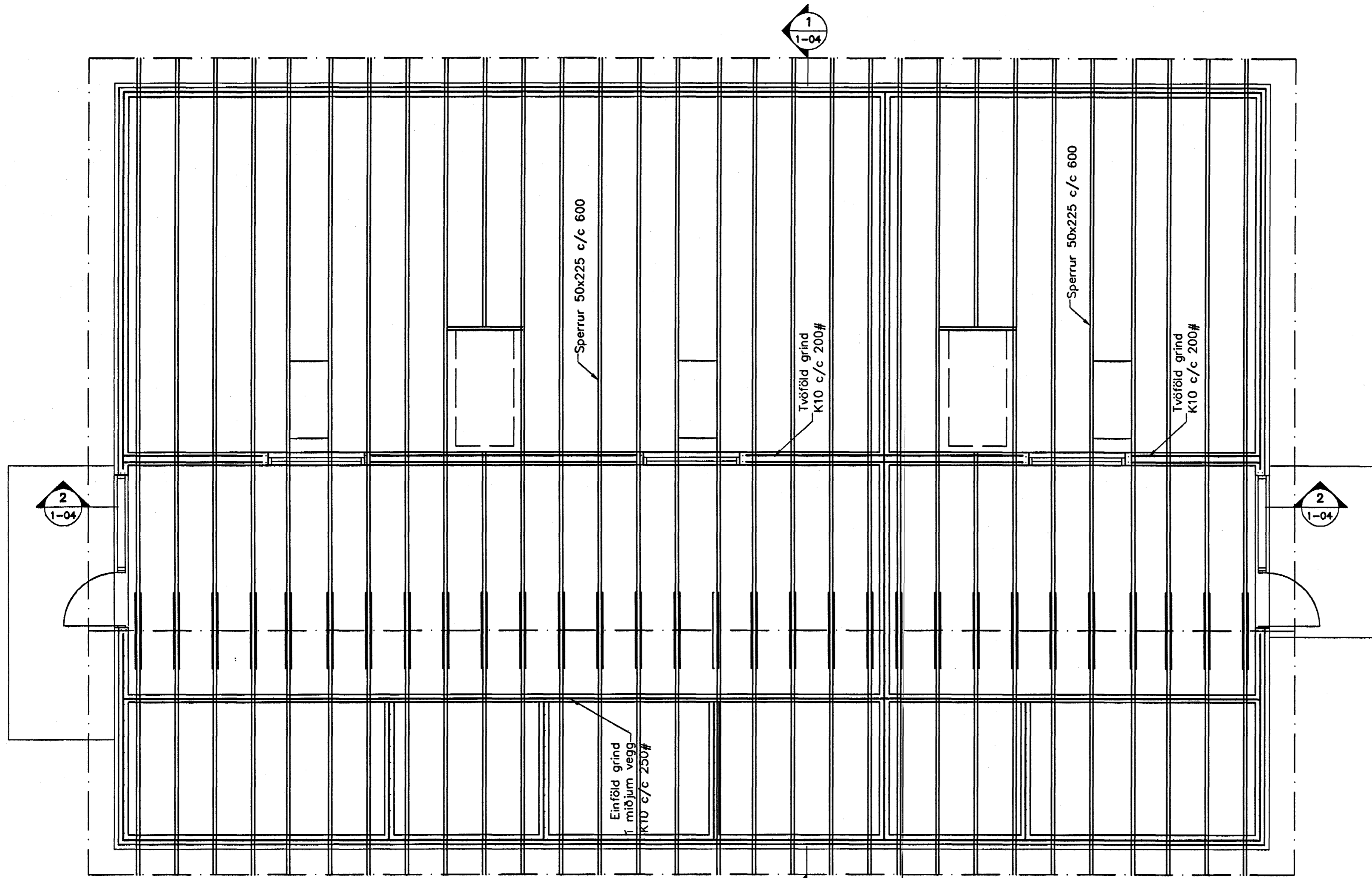
Þakvirki. Grunnmynd. 1:50
