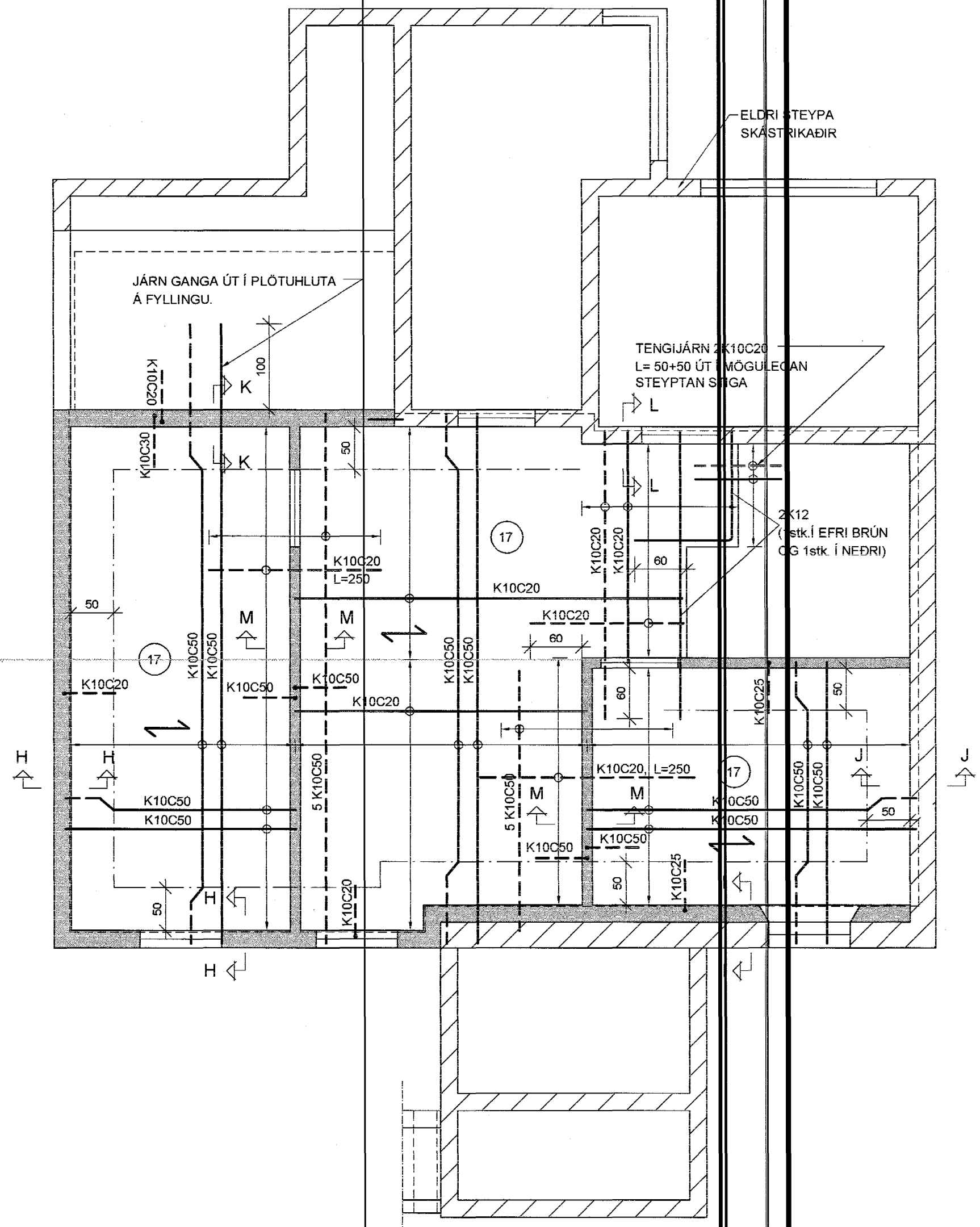
GRUNNMYND 1:50 MIÐJUHLUTI
