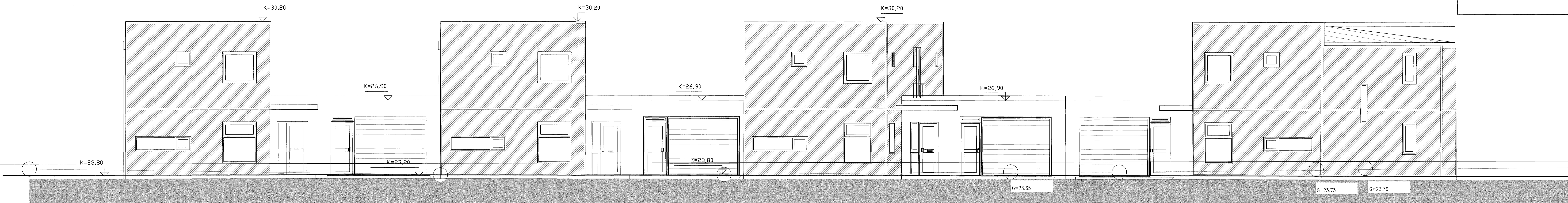
1 GRUNNMYND 1:100
