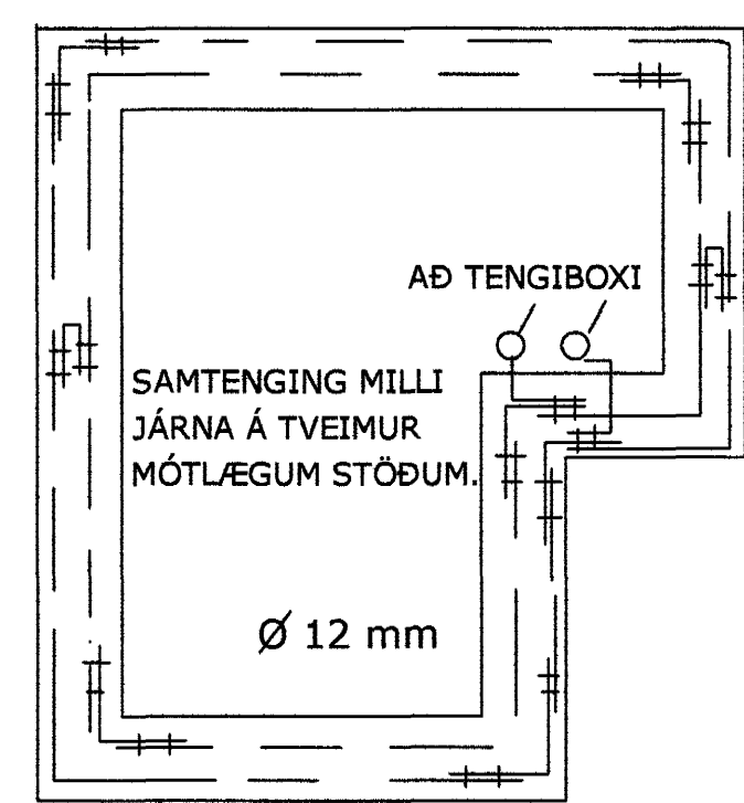
GRUNNMYND SÖKKULVEGGJA
