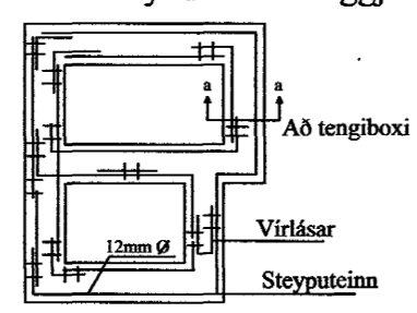
Grunnmynd sökkulveggja
