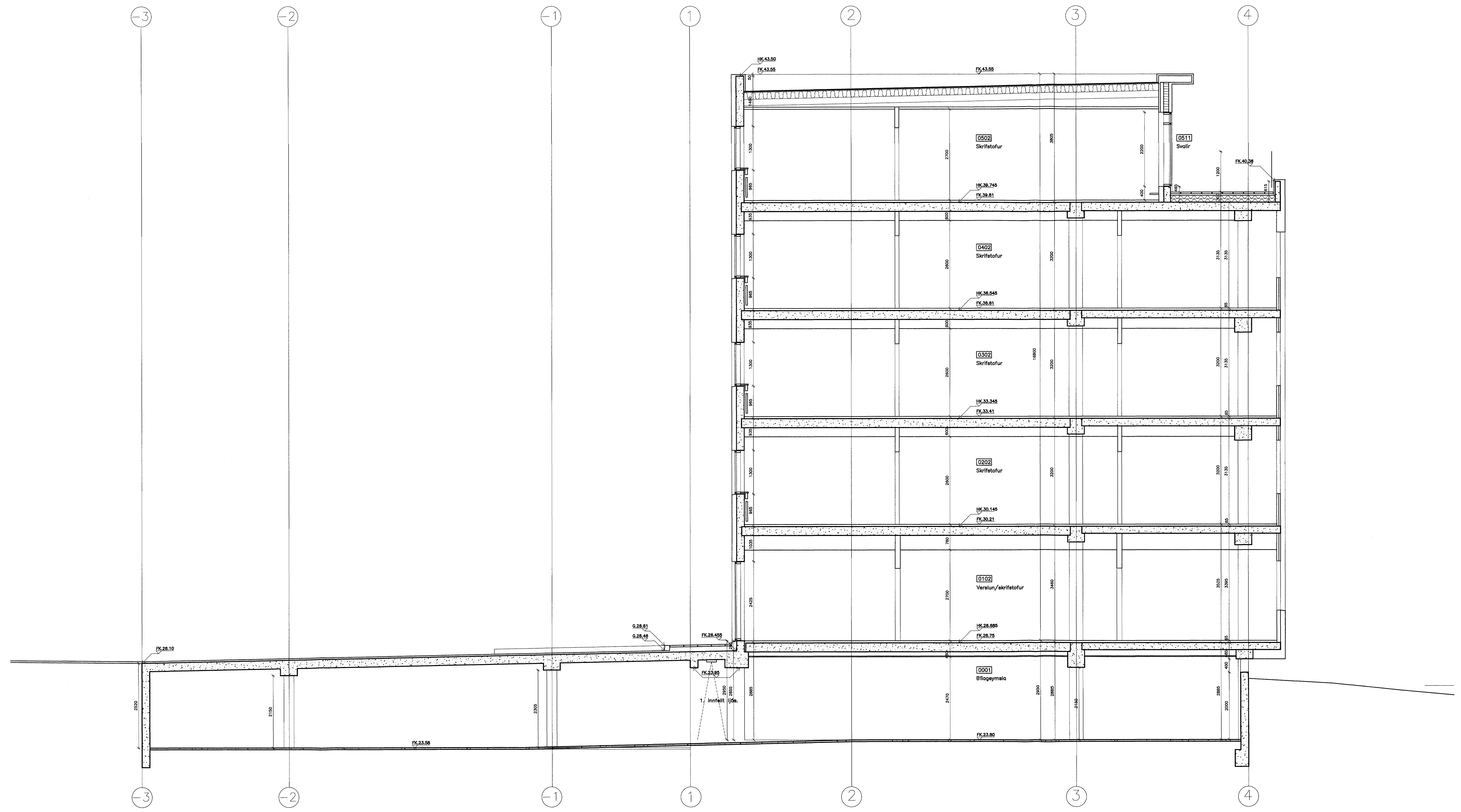
SNID A-A
