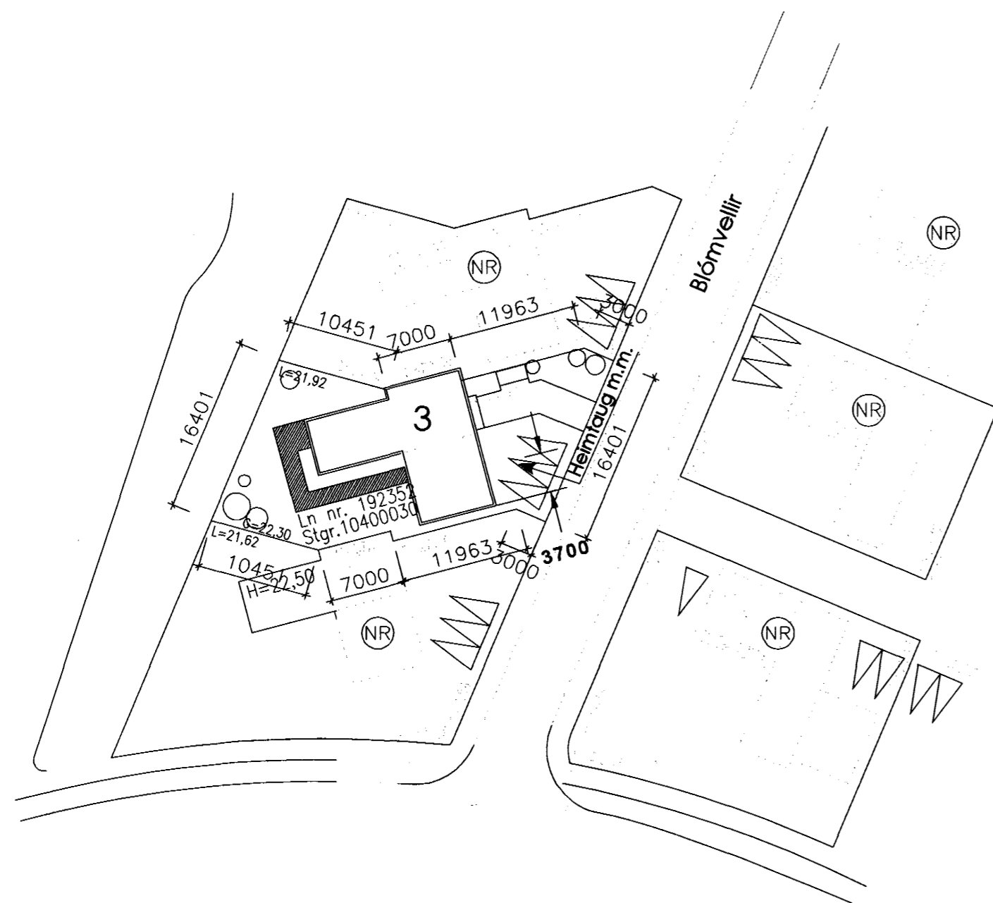
Afstöðumynd 1:500
