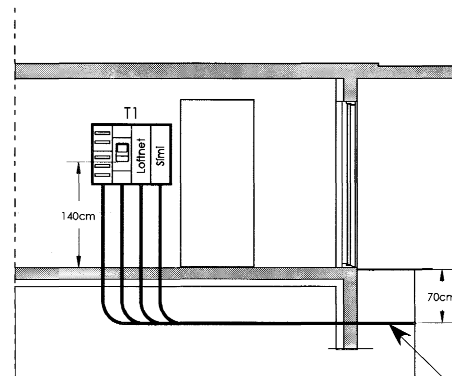
Snið 1:50
