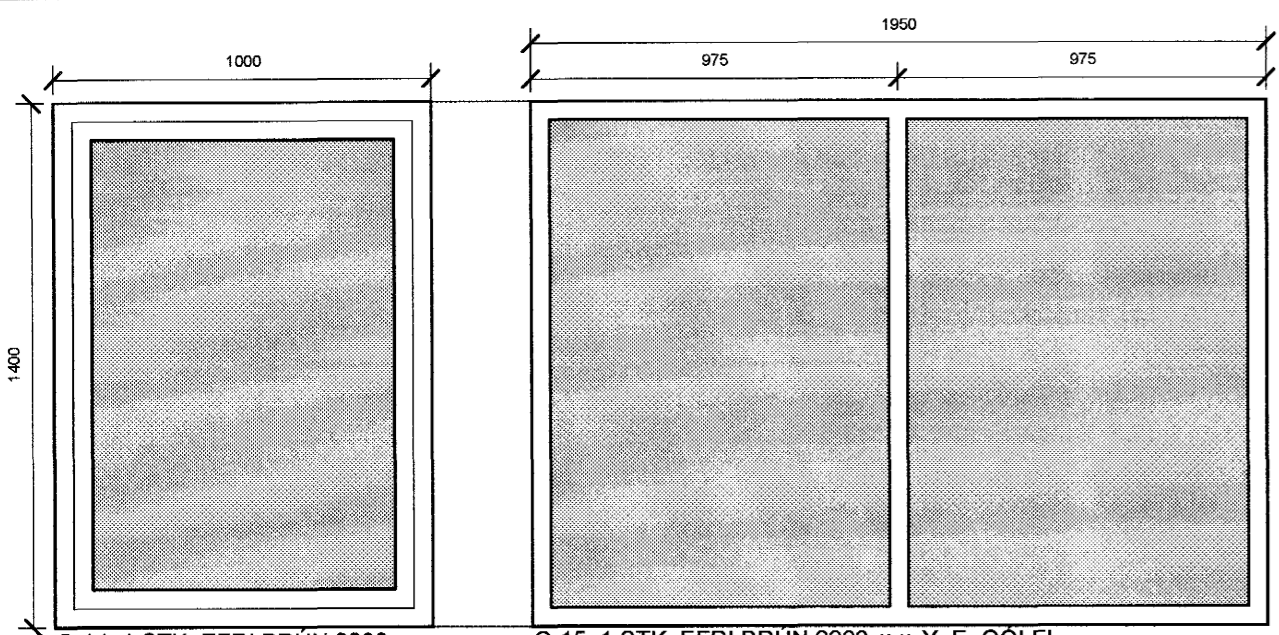
G-14, 1 STK. EFRI BRÚN 2200 mm Y. E. GÓLFI SETTUR SAMAN VIÐ G-15 SEM HORNGLUGGI
