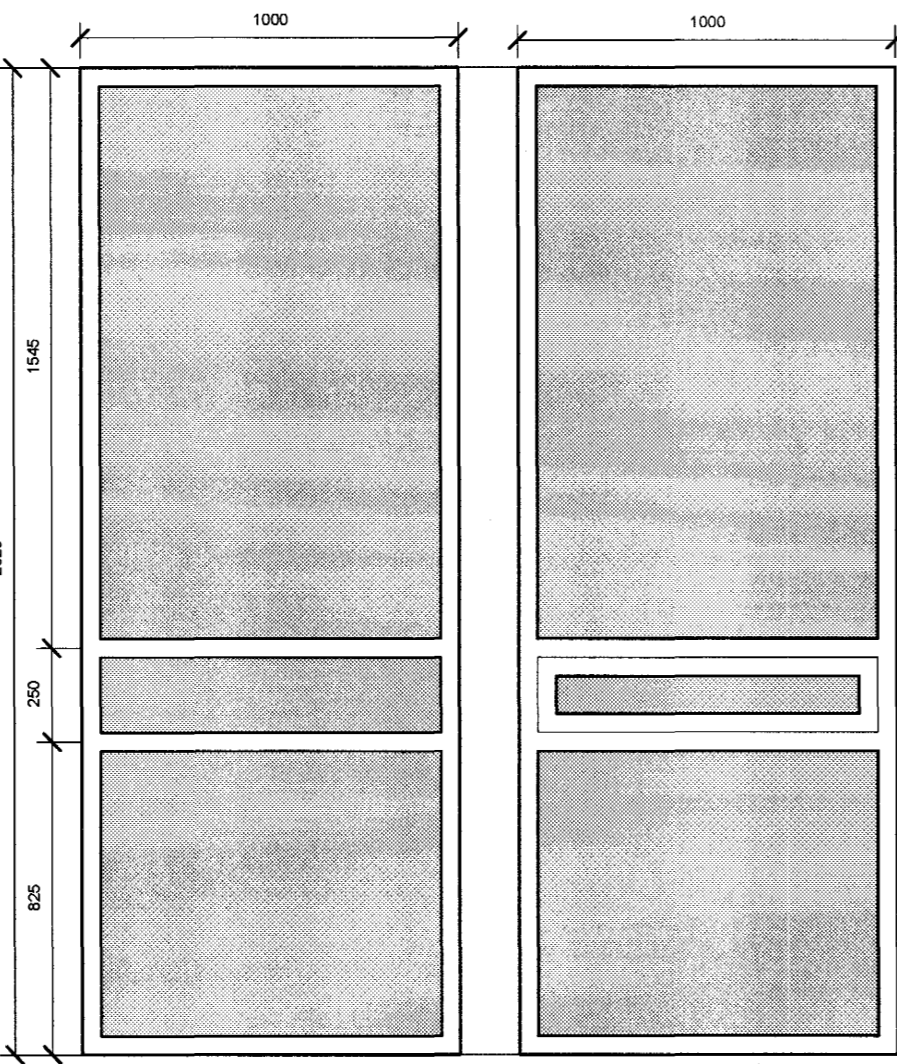
G-7, 1 STK. EFRI BRÚN 2620 mm Y. E. GÓLFI SETTUR SAMAN VIÐ G-9 SEM HORNGLUGGI
