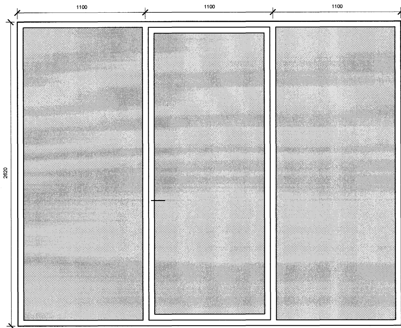
G-1, 2 STK. EFRI BRÚN 2620 mm YFIR ENDANLEGU GÓLFI. RENNIBURÐ OPNAST TIL HÆGRI Í ÖÐRUM EN VINSTRI Í HINUM
