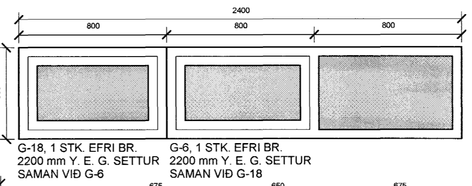
G-12, 1 STK. EFRI BRÚN 2200 mm Y. E. GÓLFI SETTUR SAMAN VIÐ G-13 SEM HORNGLUGGI
