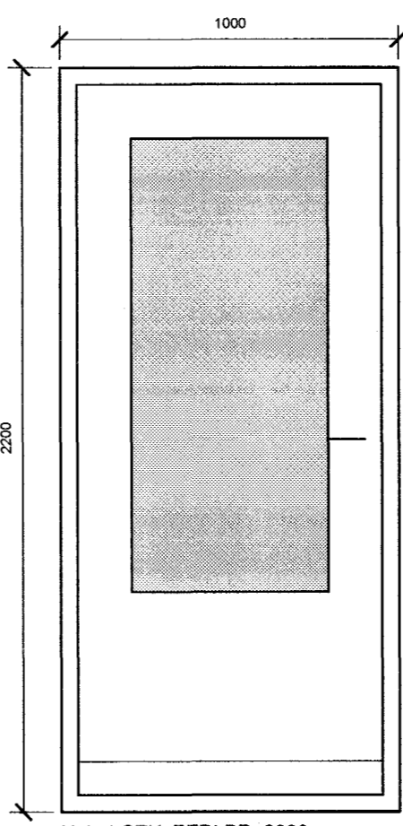
H-1, 1 STK. EFRI BR. 2200 mm YFIR ENDANLEGU GÓLFI
