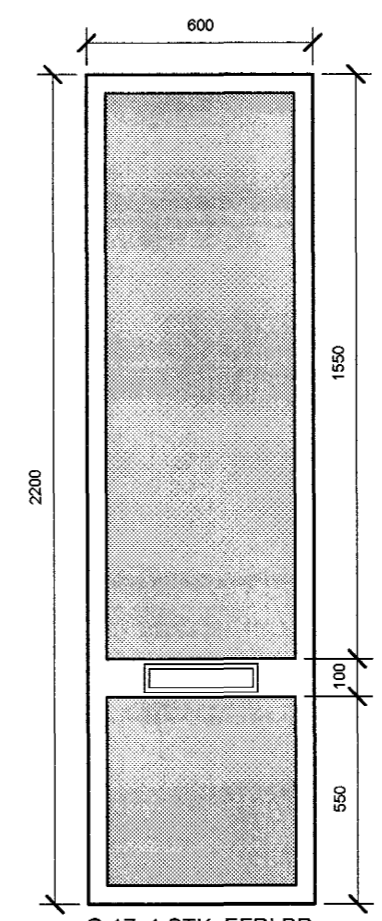
G-17, 1 STK. EFRI BR. 2200 mm Y. E. G.
