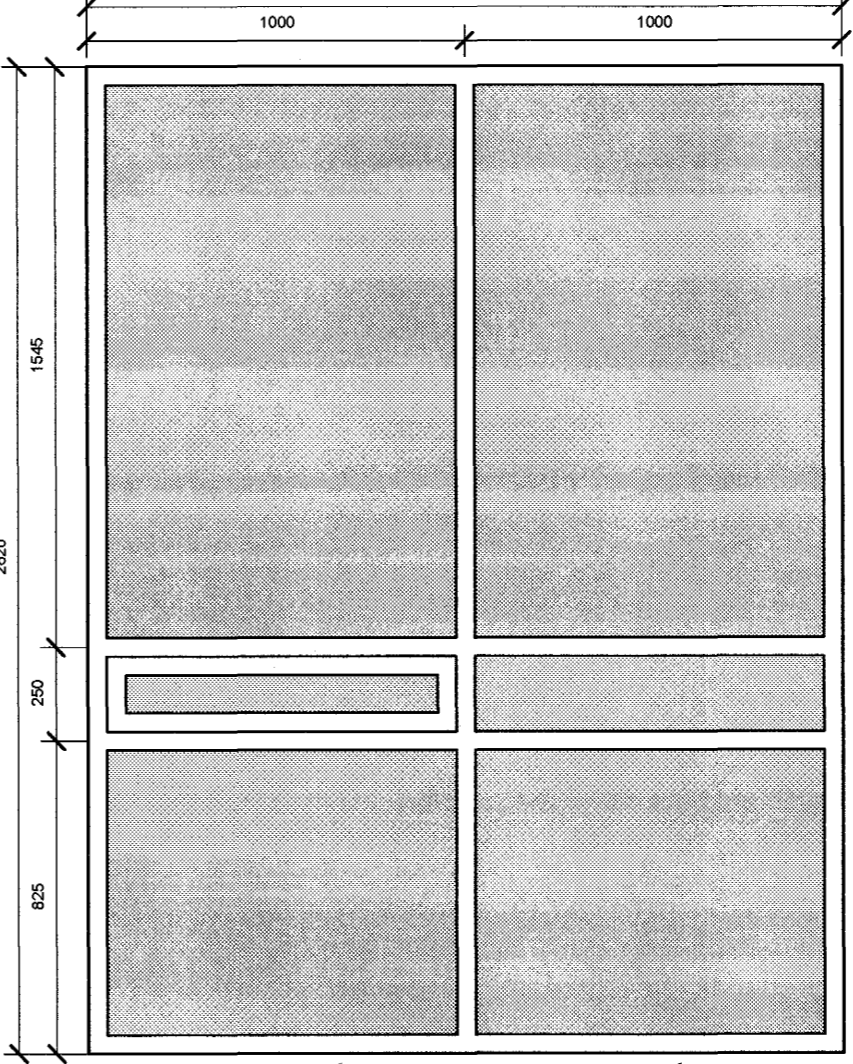
G-16, 1 STK. EFRI BRÚN 2620 mm YFIR ENDANL. GÓLFI
