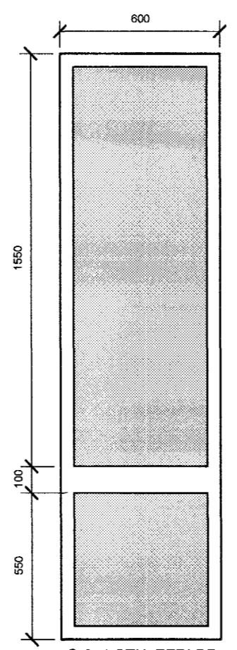
G-3, 1 STK. EFRI BR. 2200 mm Y. E. G.
