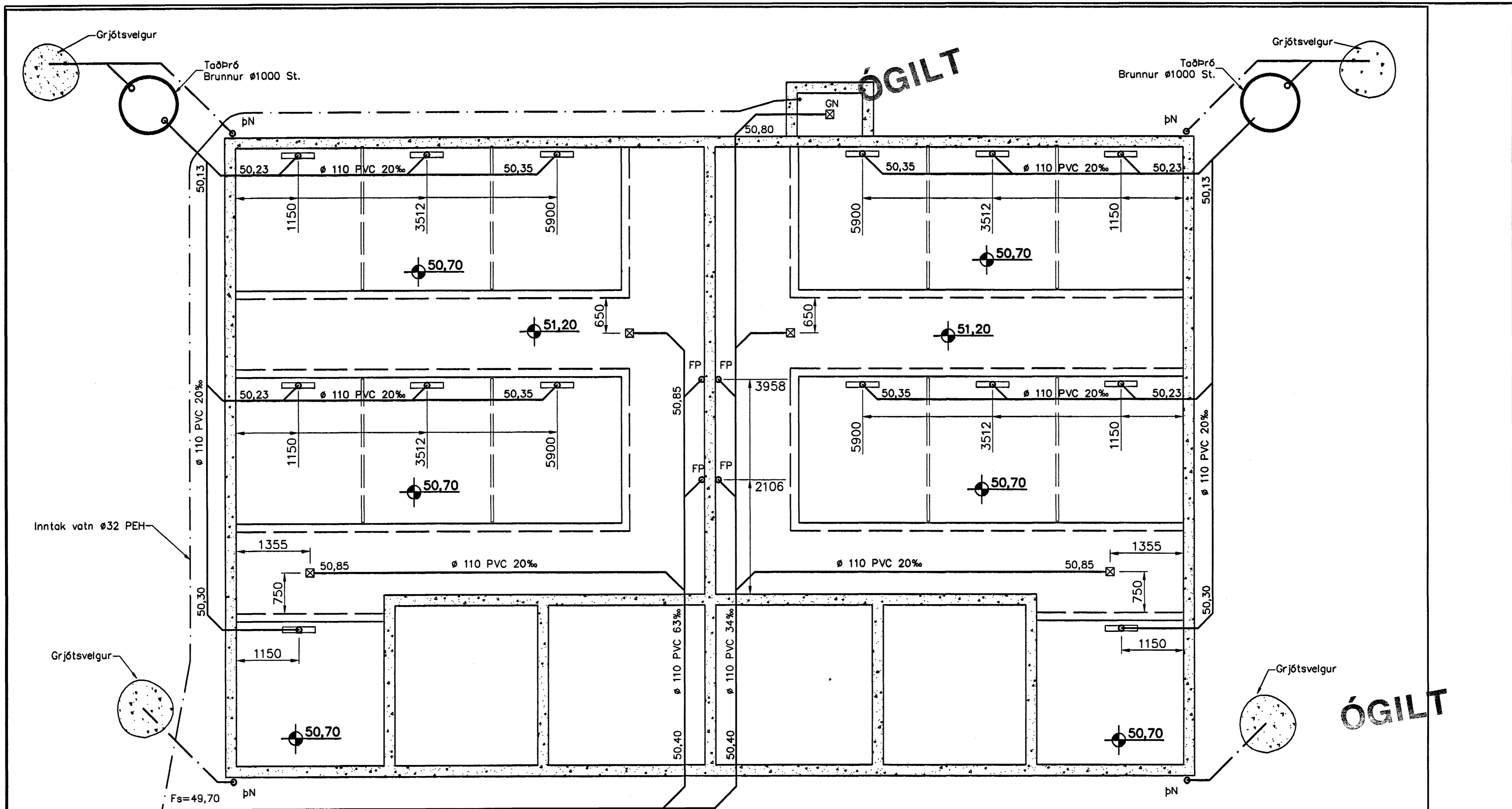
Grunnlagnir. Grunnmynd. 1:50
