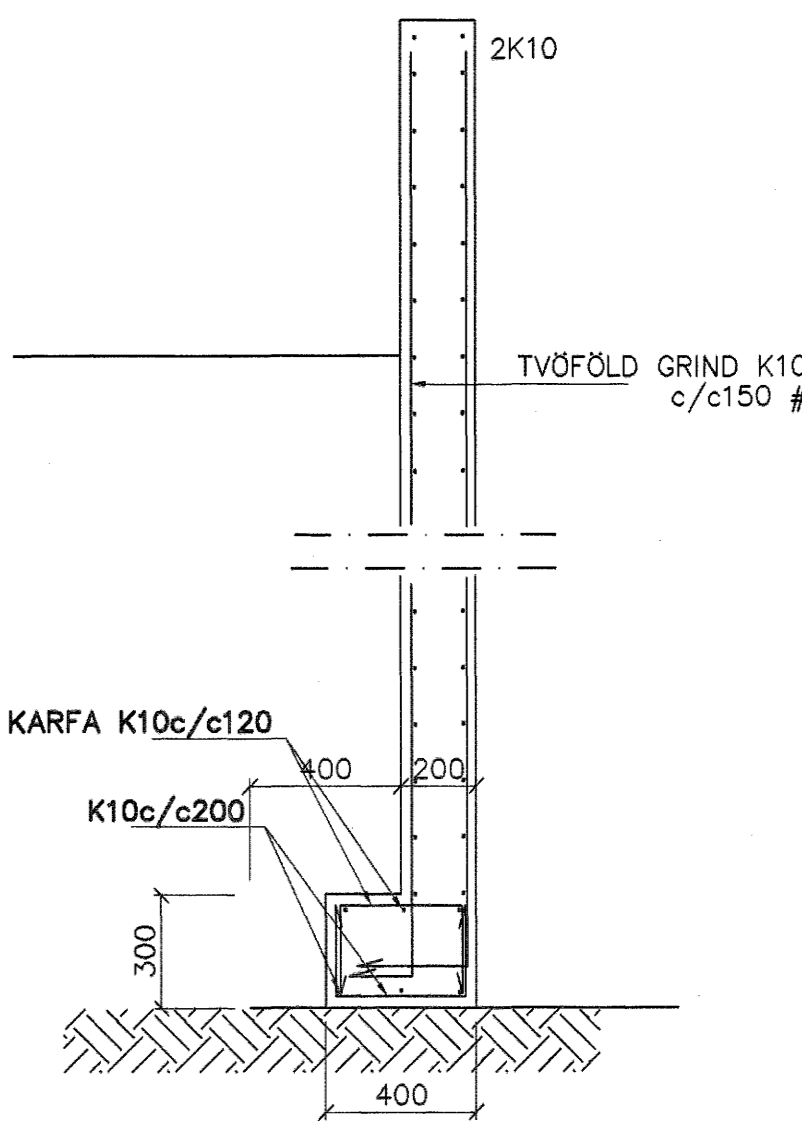
SNÍÐ 15 1:20
