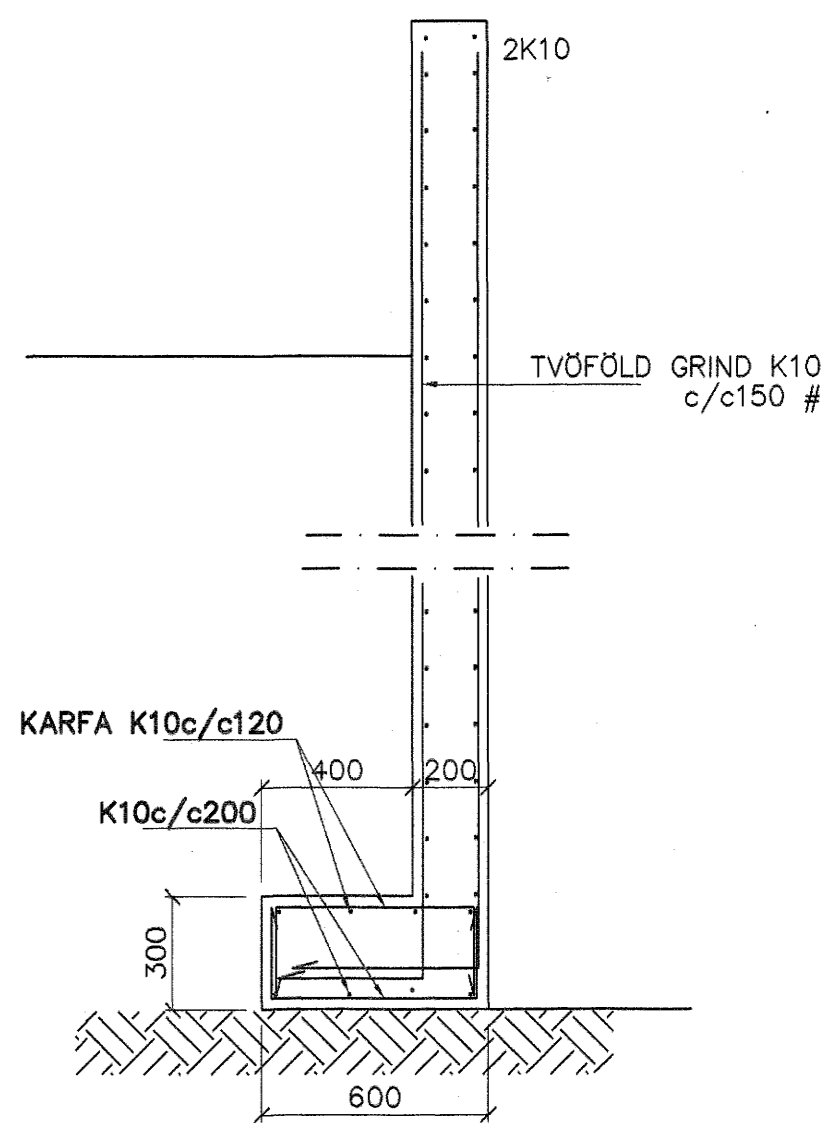
SNÍÐ 14 1:20
