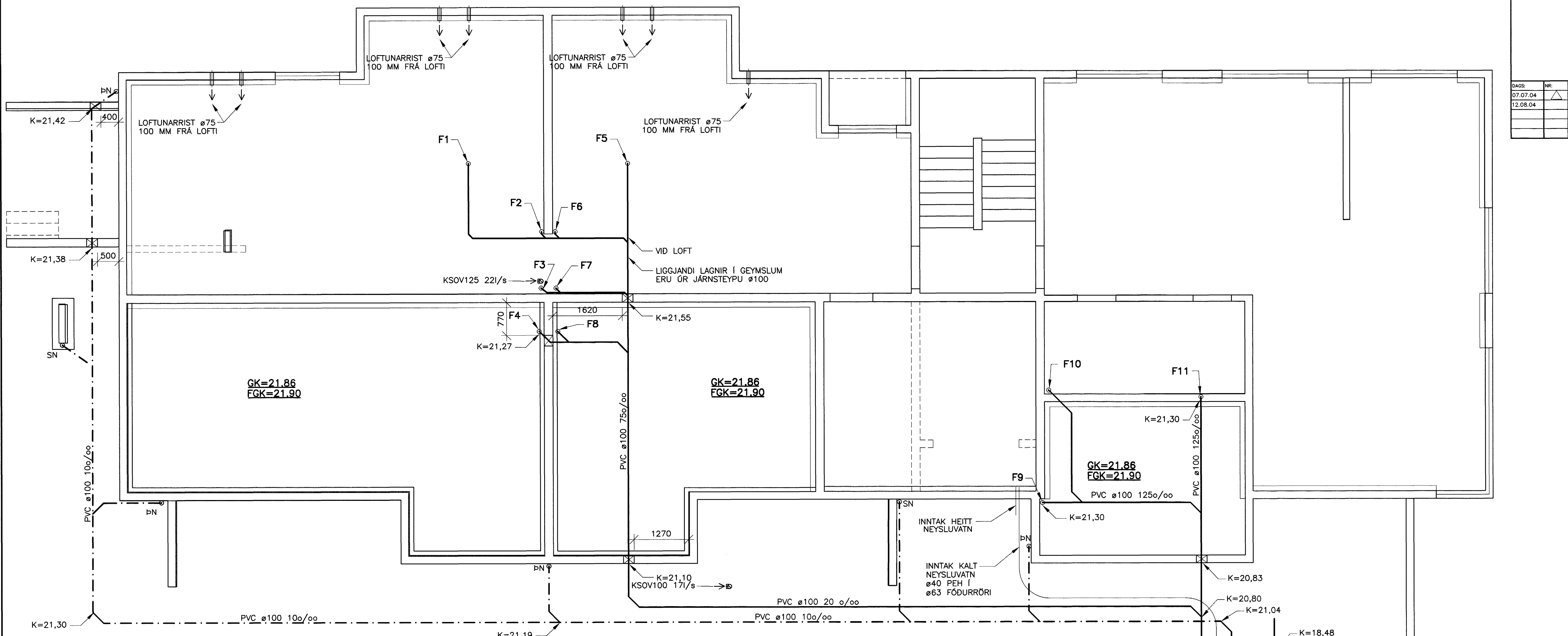
GRUNNLAGNIR GRUNNMYND. 1:50
