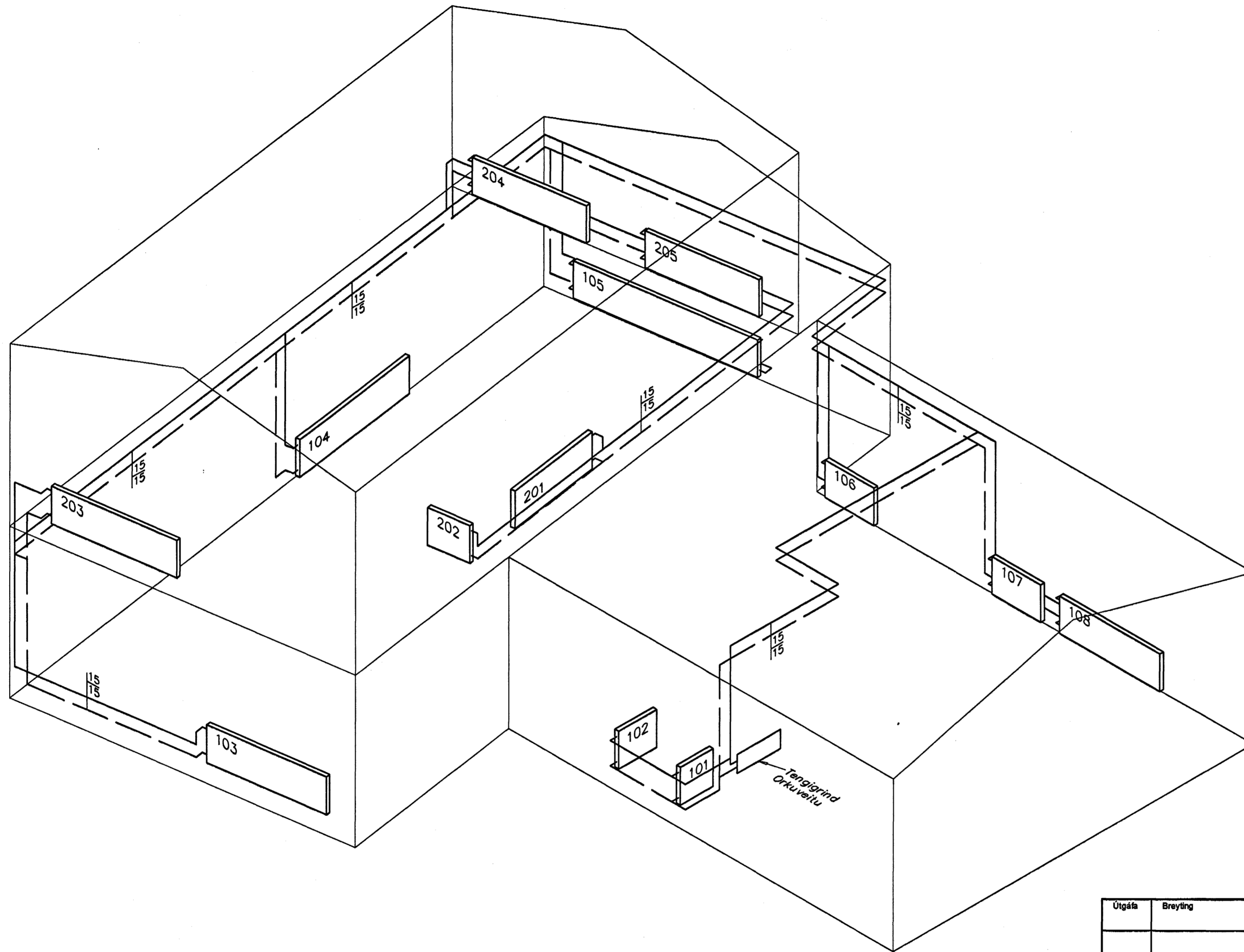
Hitalagnir, Rúmmynd, 1:50
