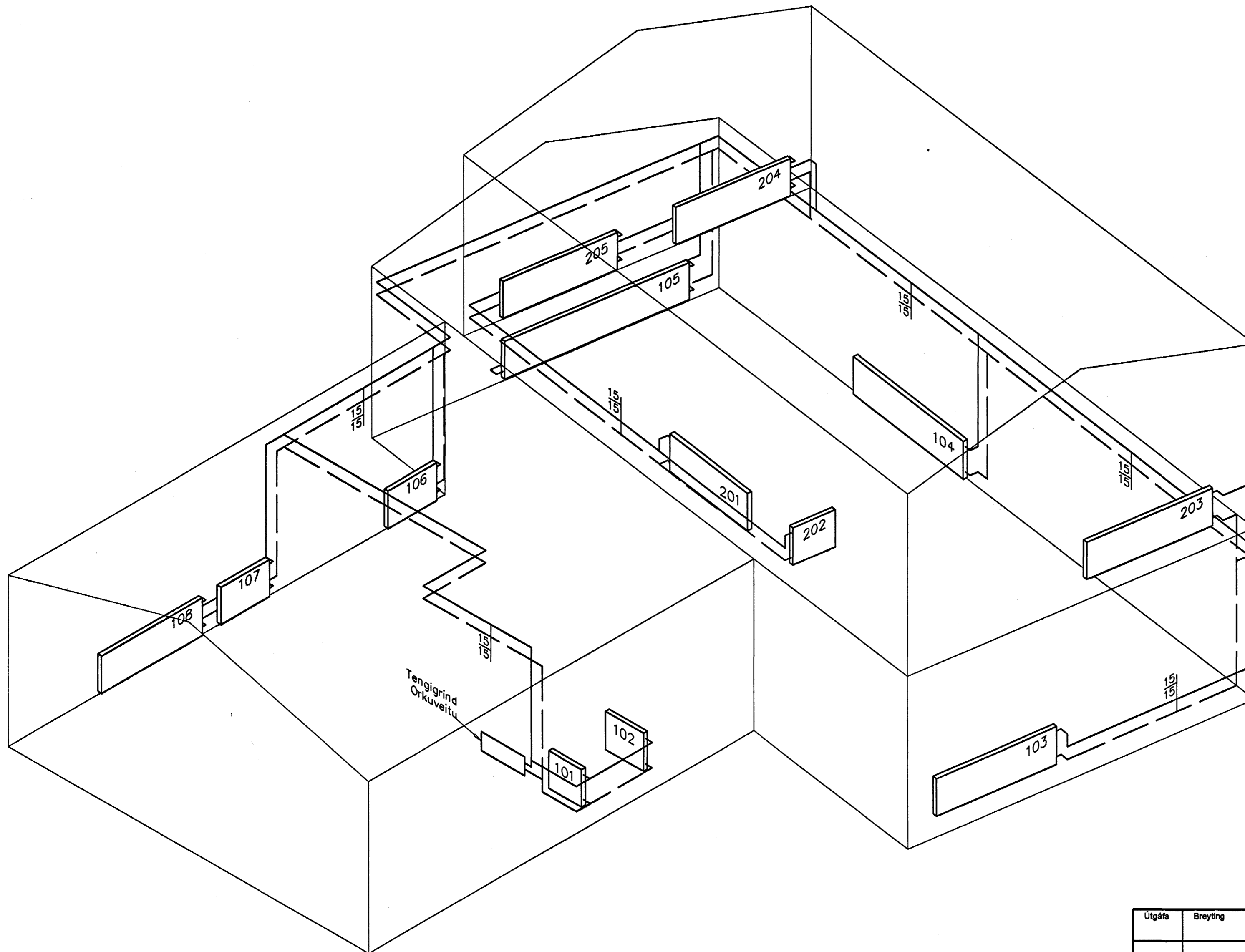
Hitalagnir, Rúmmynd, 1:50
