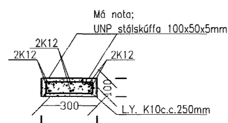
Súla S1 1:20
