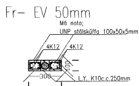
Súla S2 1:20
