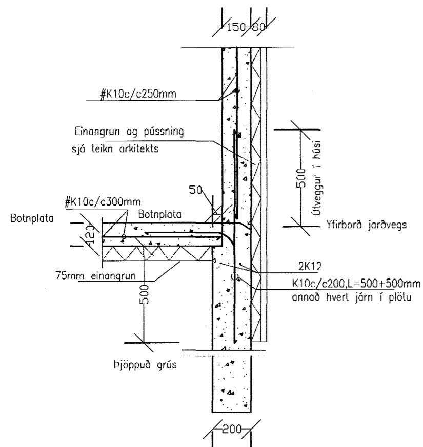
Snið A1 1:20
