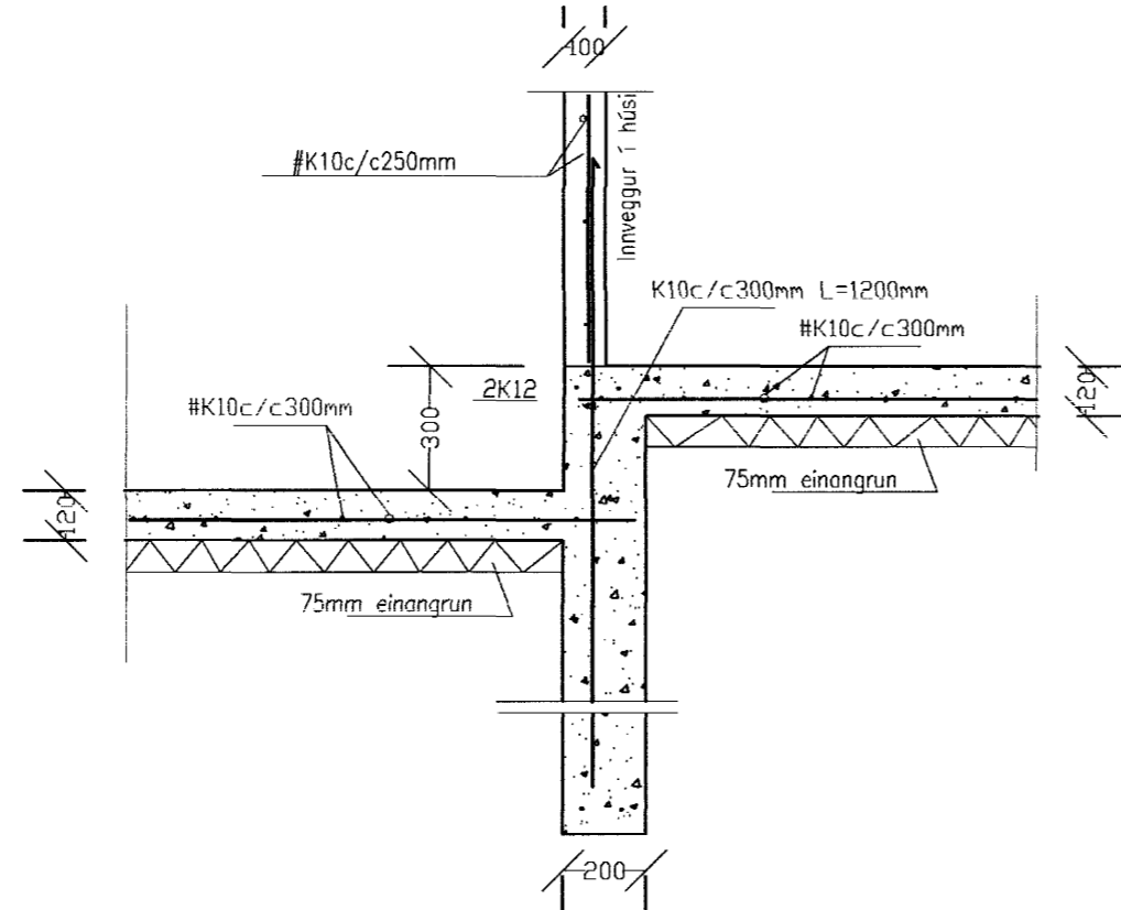
Snið A2 1:20
