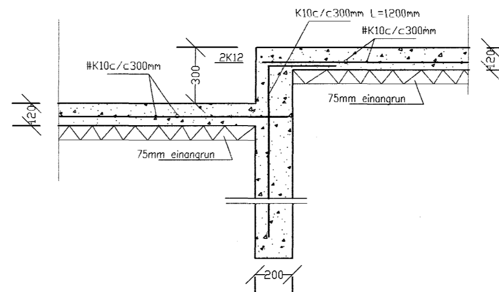
Snið A21 1:20
