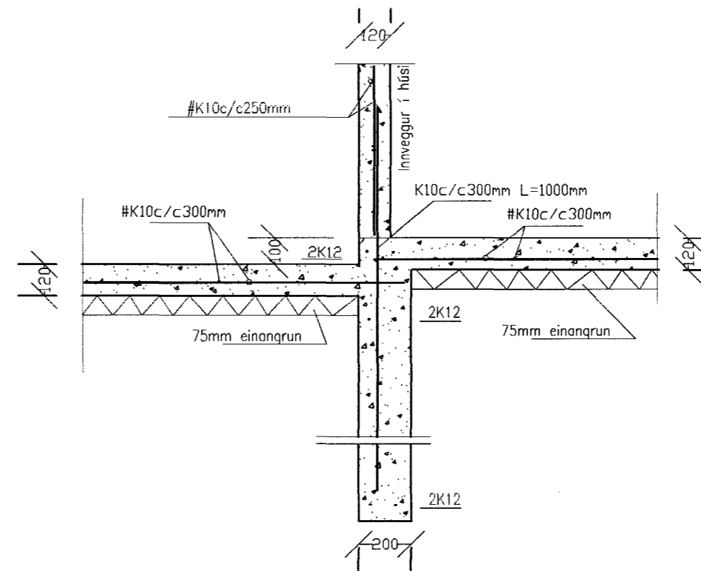
Snið A4 1:20
