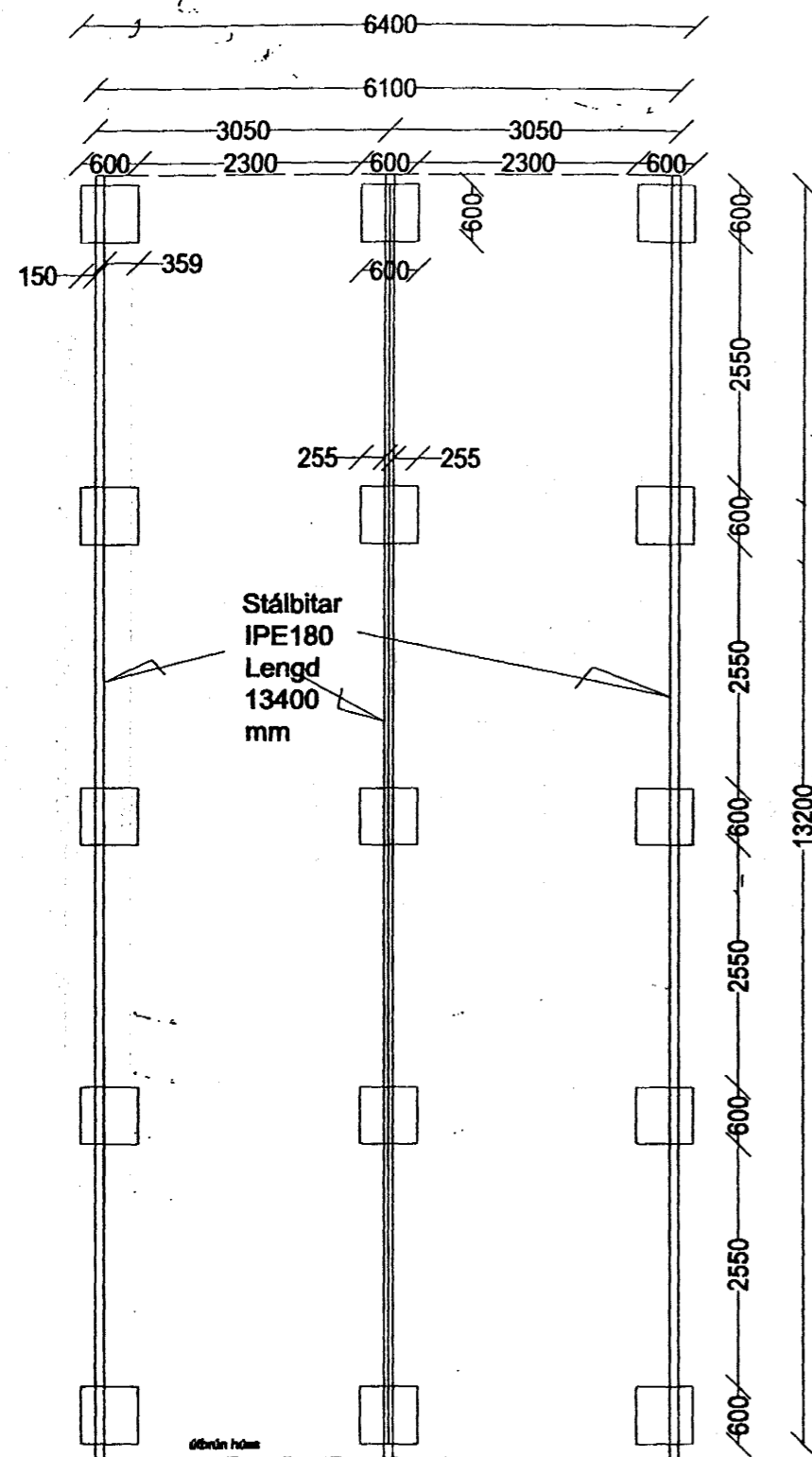
Grunnmynd undirstaðna 1:50
