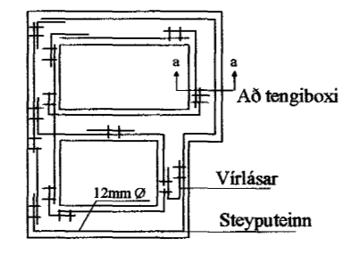
Grunnmynd sökkulveggja
