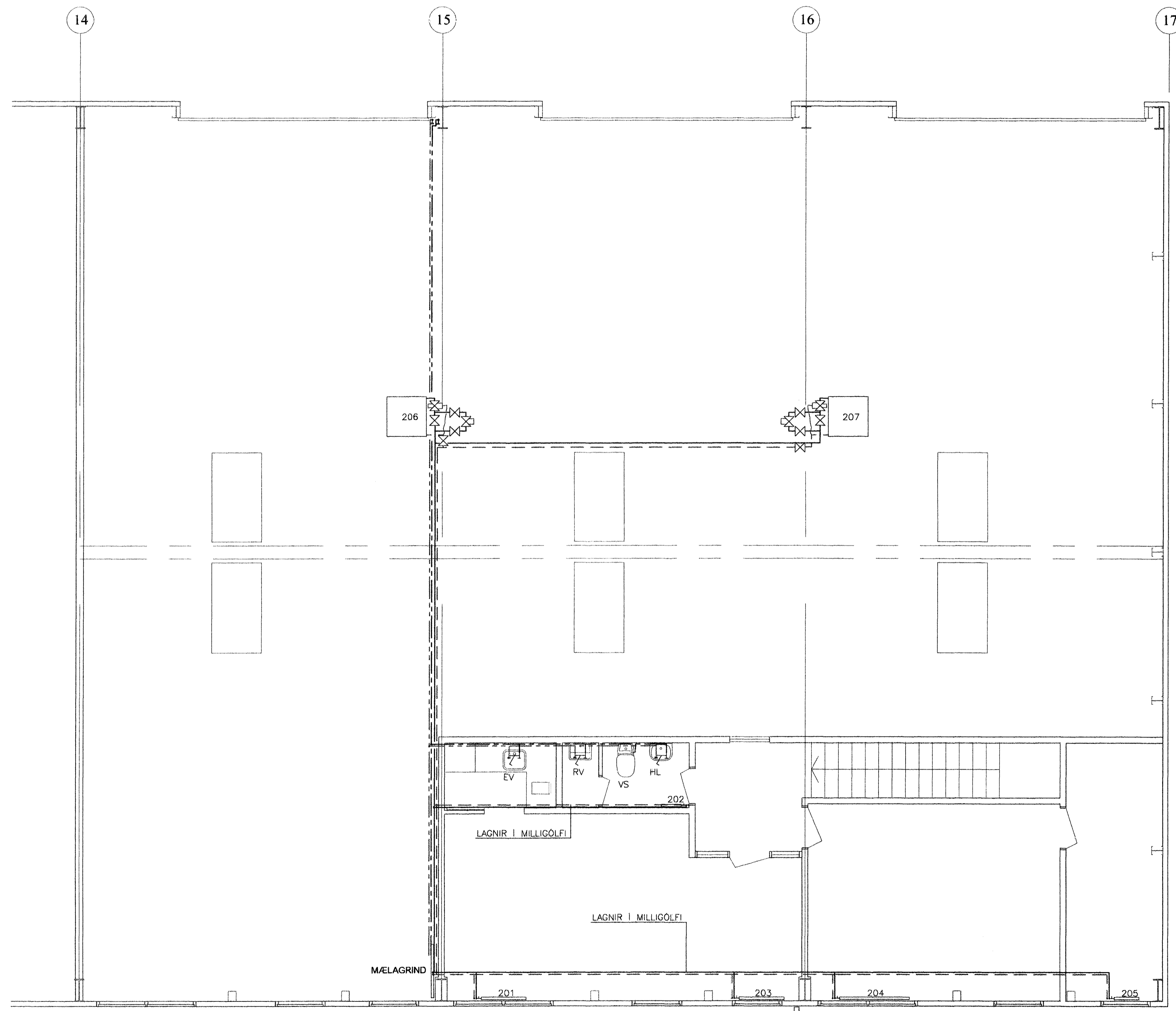
GRUNNMYND 2. HÆÐ
