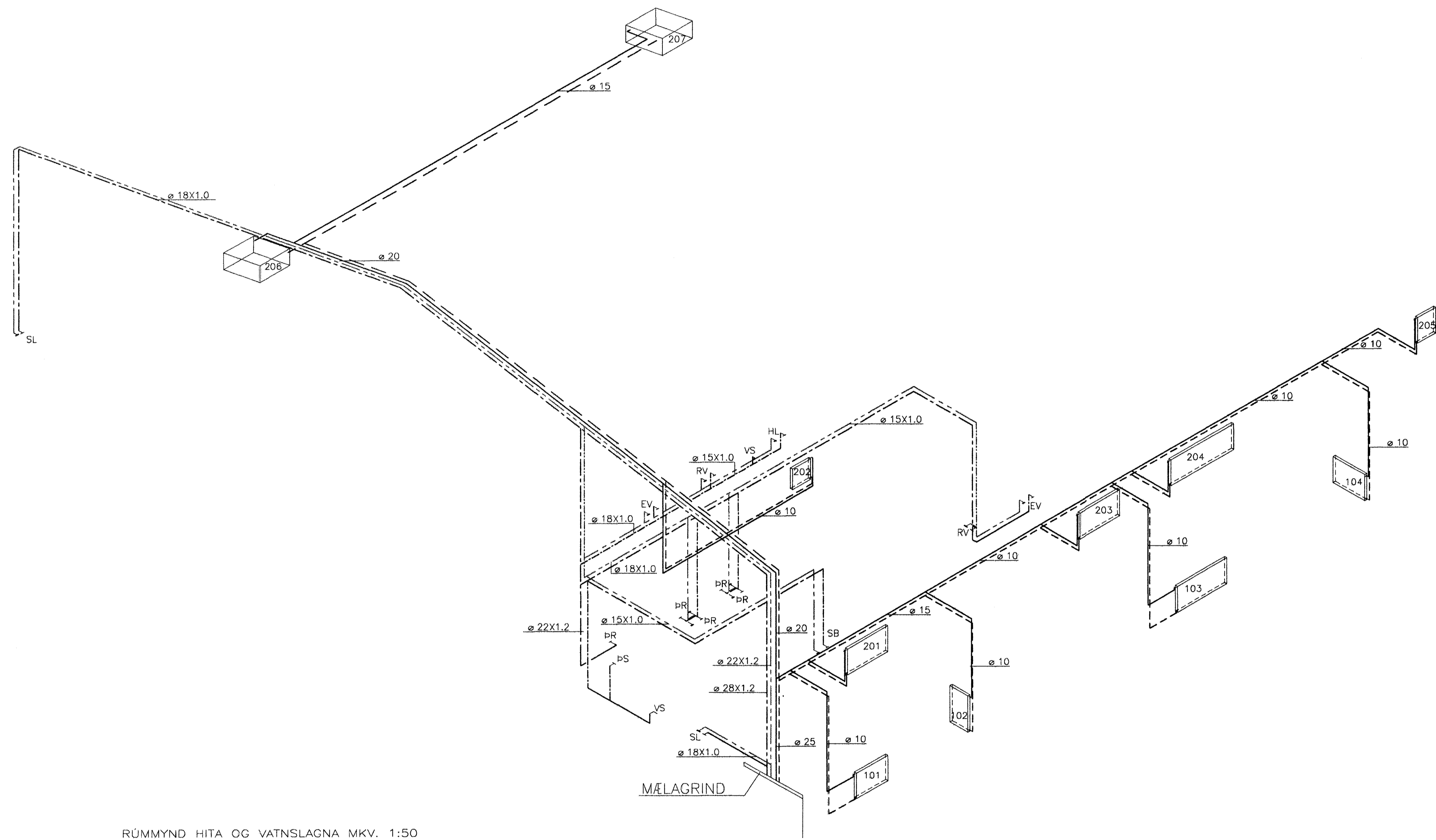
RÚMMYND HITA OG VATNSLAGNA MKV. 1:50
