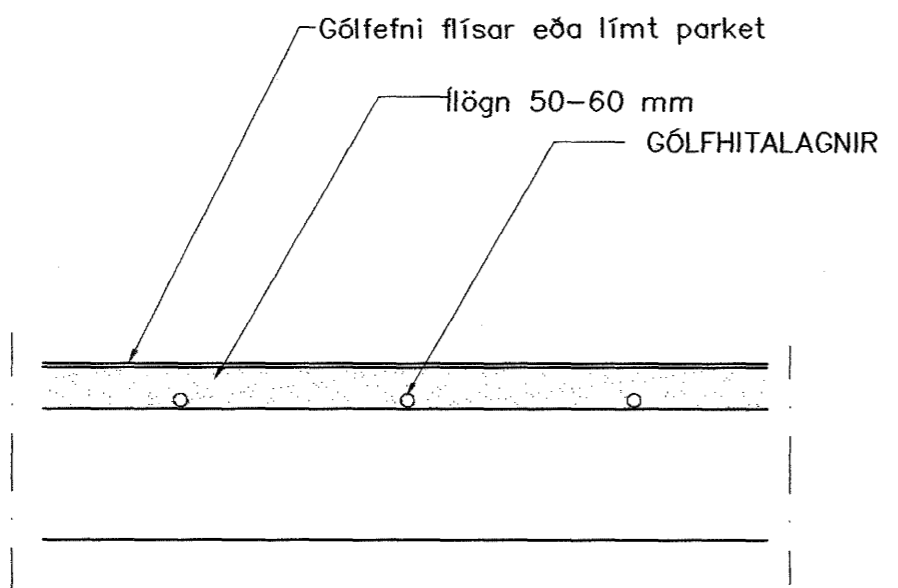
GÓLFHITALAGNIR SNIÐ 1:20
