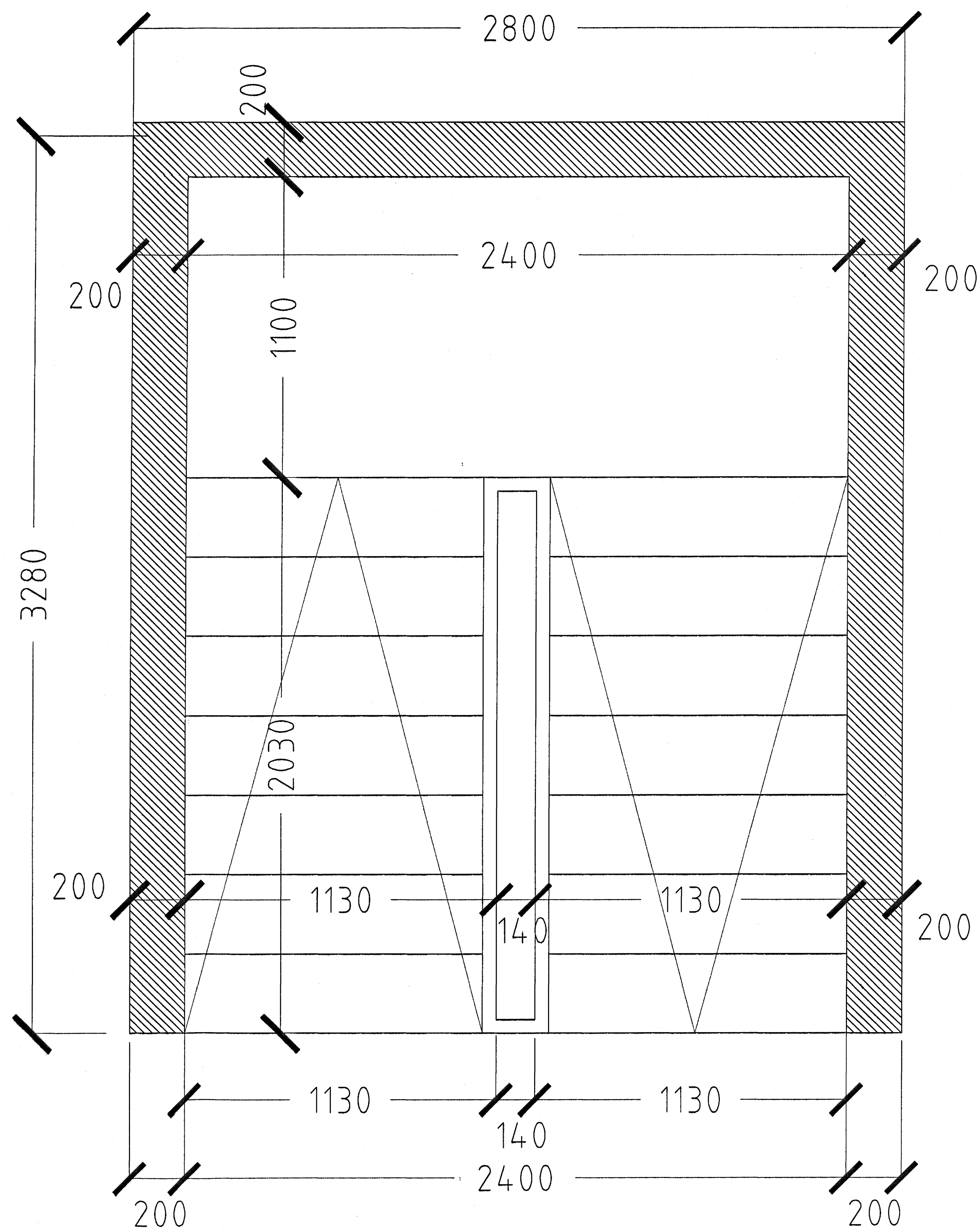
GRUNNMYND STIGI MKV. 1:10. HÚS 4A. MHL. 01.
