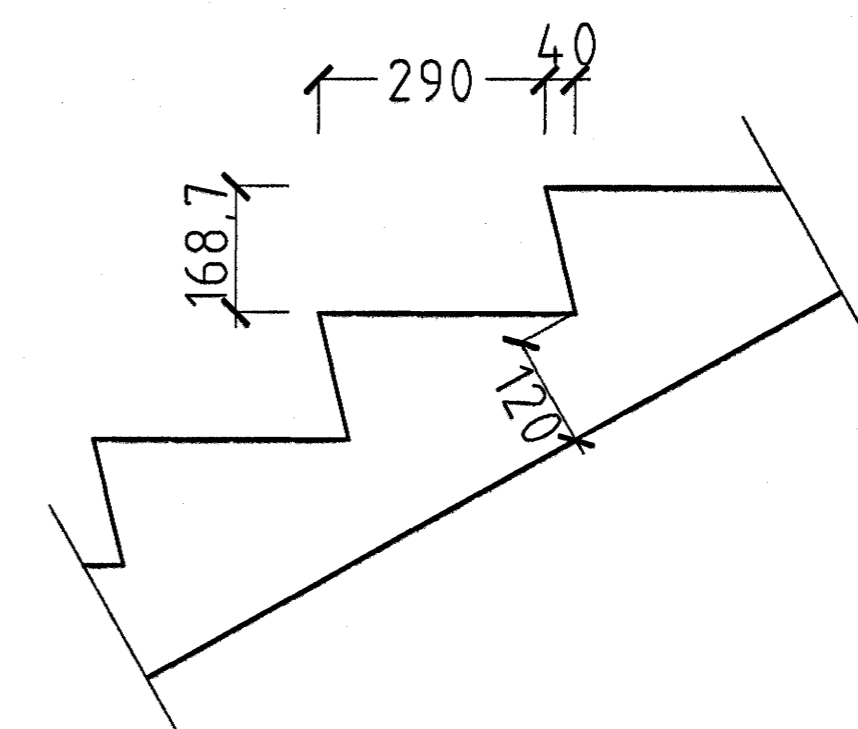
SNÍÐ Í ÞREP MKV. 1:10.
