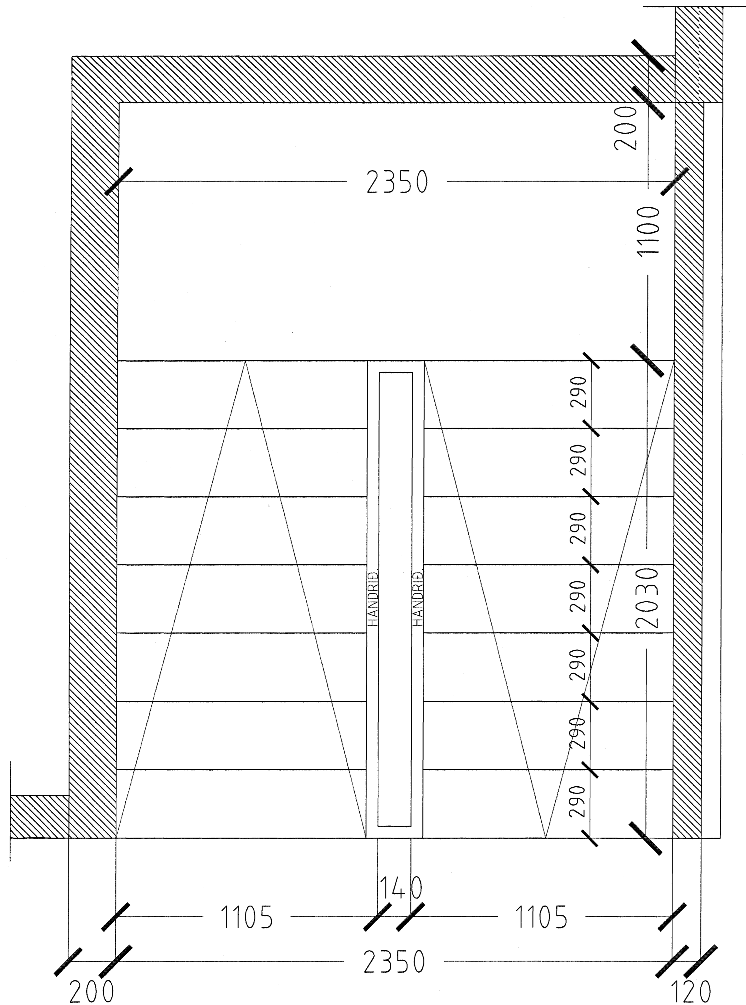
GRUNNMYND STIGI MKV. 1:10.
