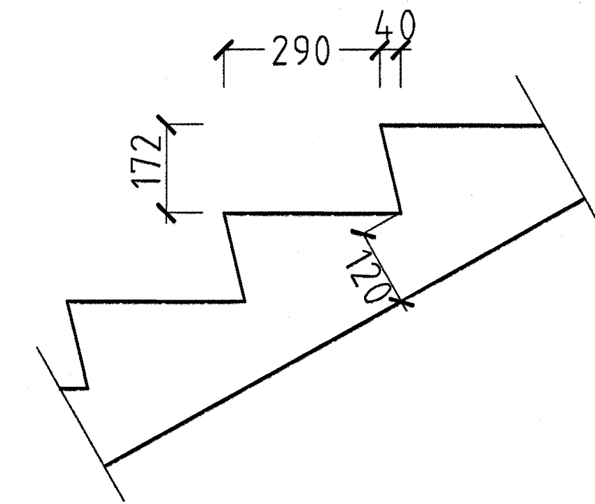
SNIÐ Í ÞREP MKV. 1:10.
