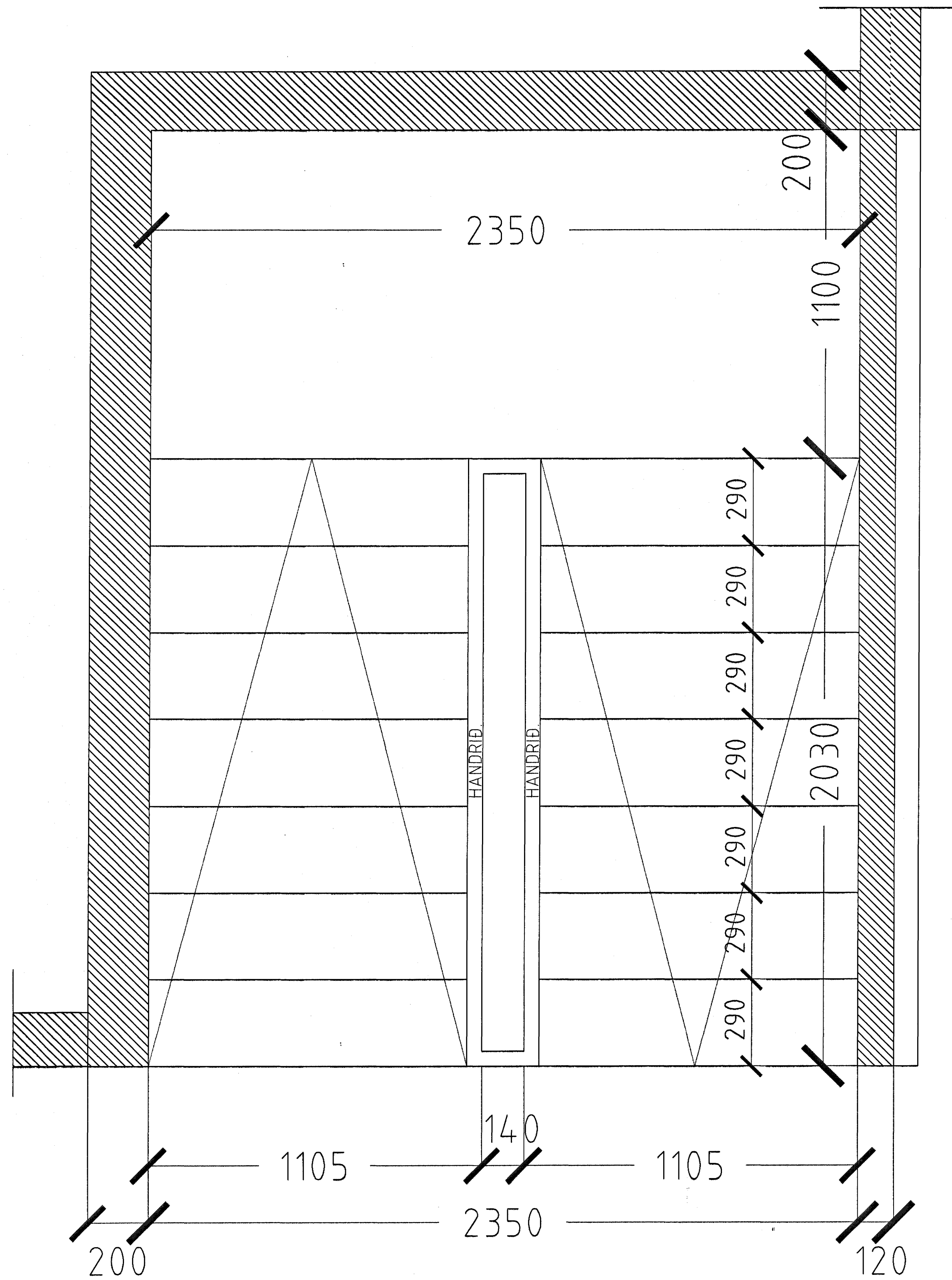
GRUNNMYND STIGI MKV. 1:10. HÚS 4B. MHL. 02.
