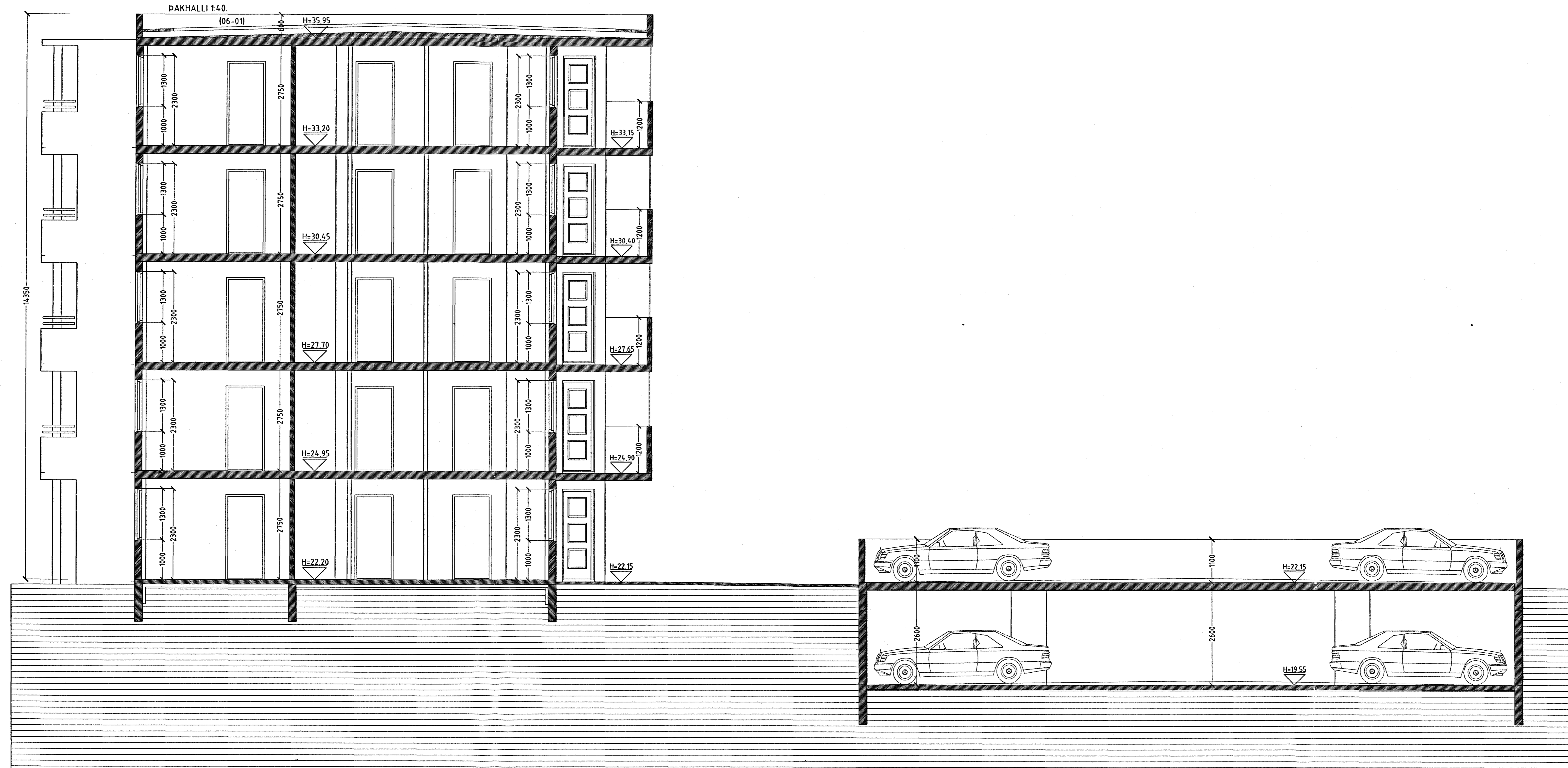
SNID A-A MKV. 1:50.
